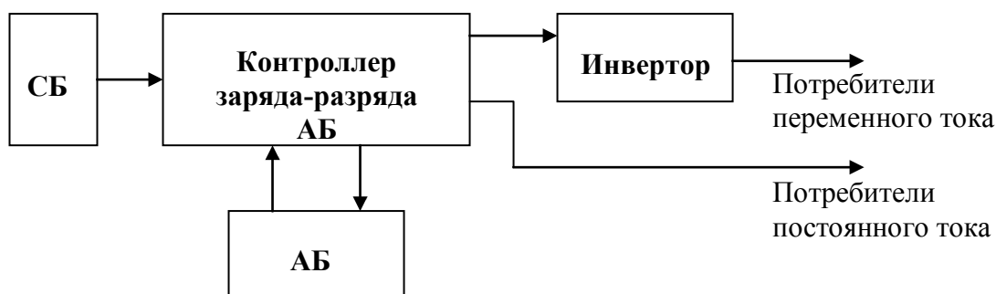
Рис. 1. Структурная схема автономной ФЭС
