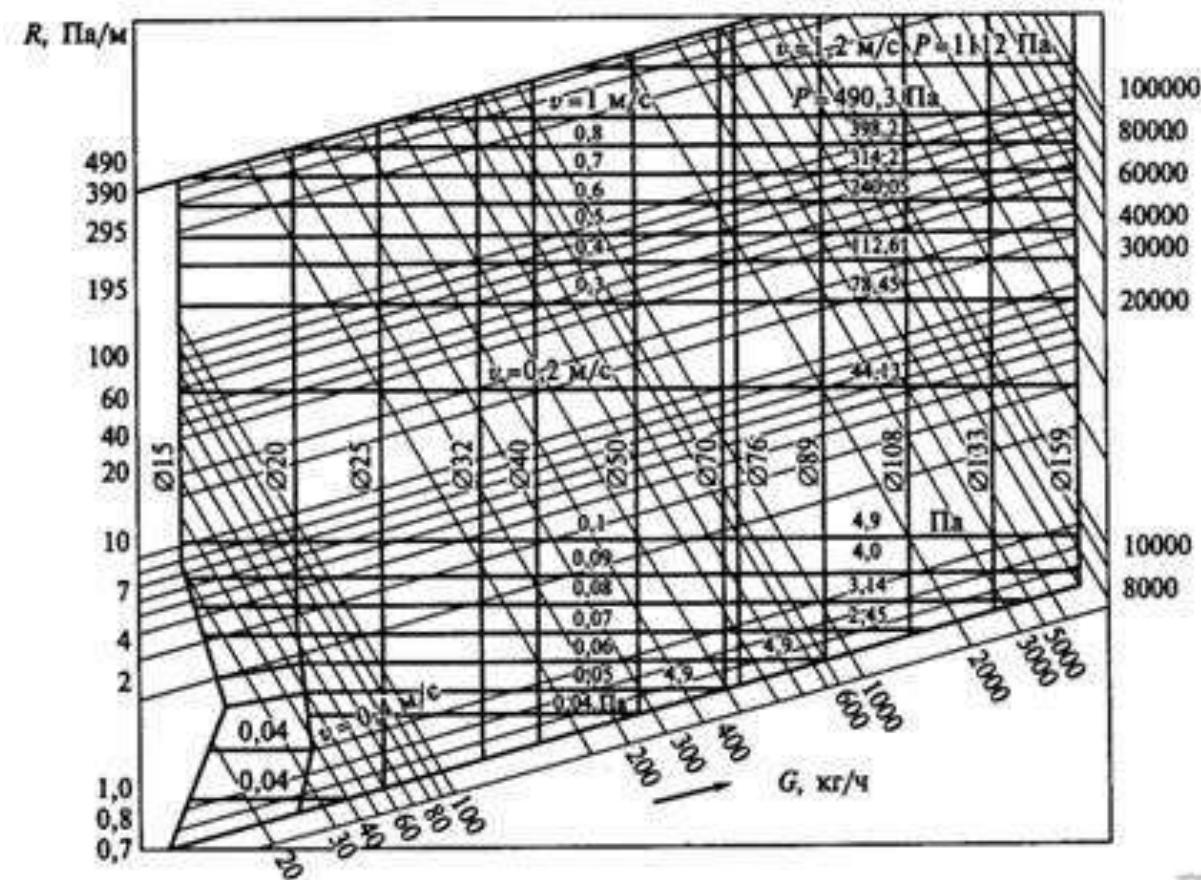
Рис. 4.1. Номограмма для расчета диаметров трубопроводов систем отопления при температуре воды 95... 70°C
