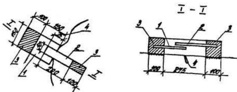
Рис. 3. Пластинчатый маяк из двух окрашенных пластинок
