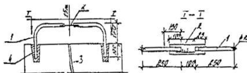
Рис. 4. Щелемер конструкции ЛенГИДЕПА
