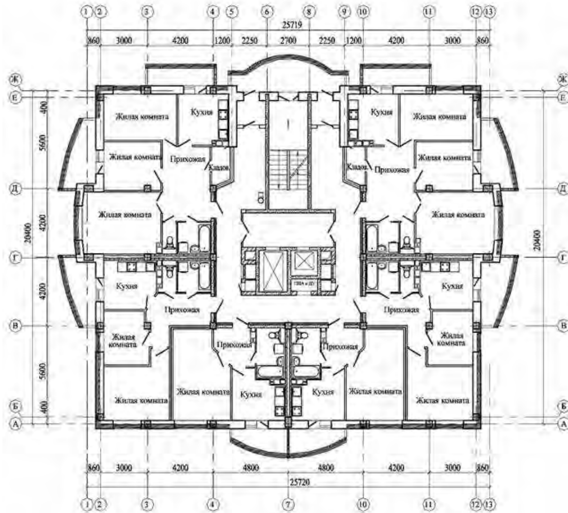
Планировка №9
