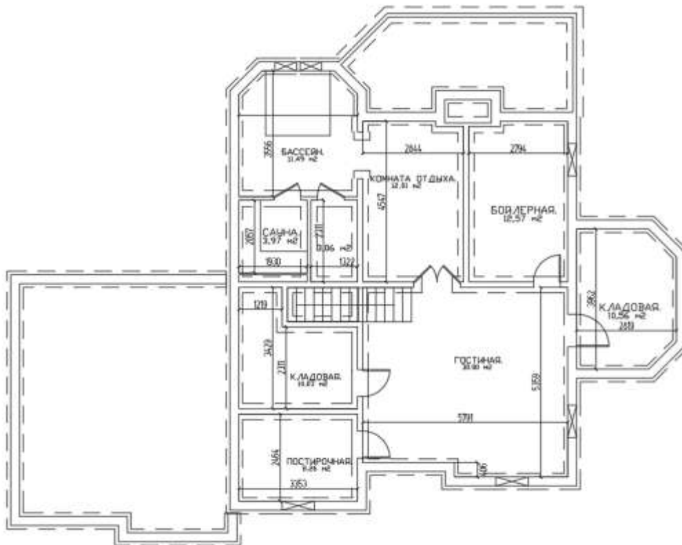
Планировка №20
