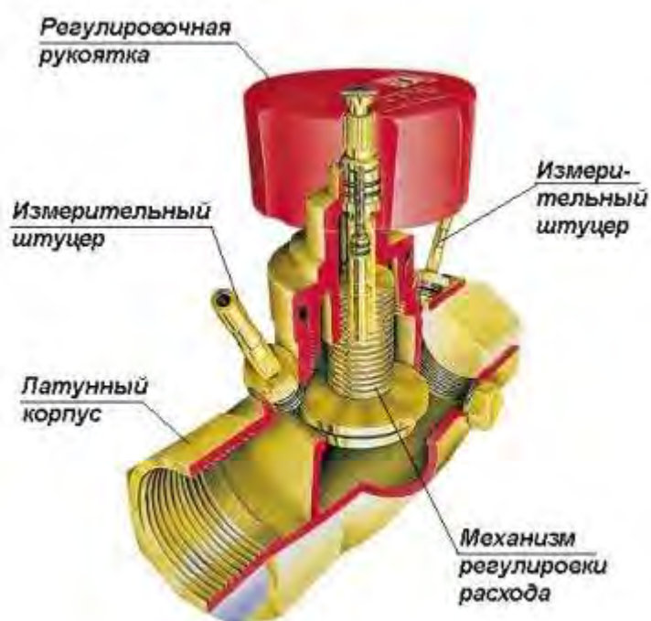
Рис. 3.10 - Балансировочный клапан
