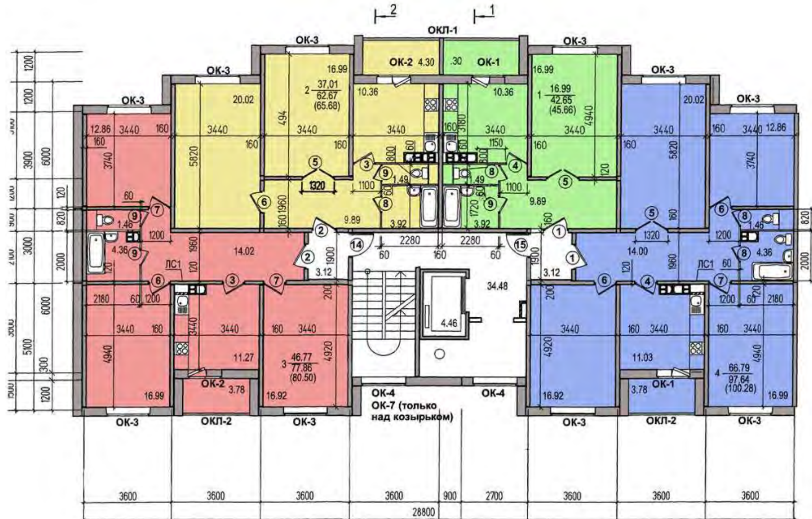
Планировка №1
