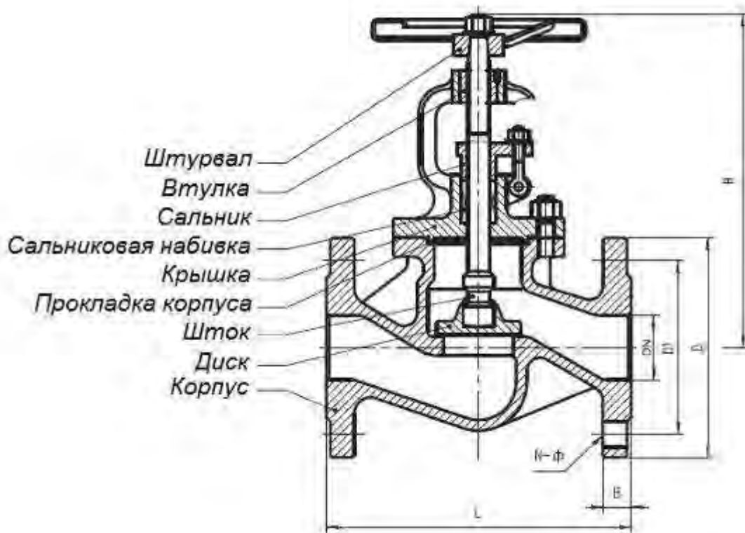
Рис. 3.3. Запорный вентиль
