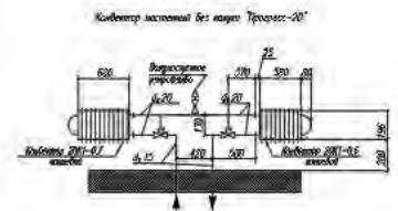
Узел Б
