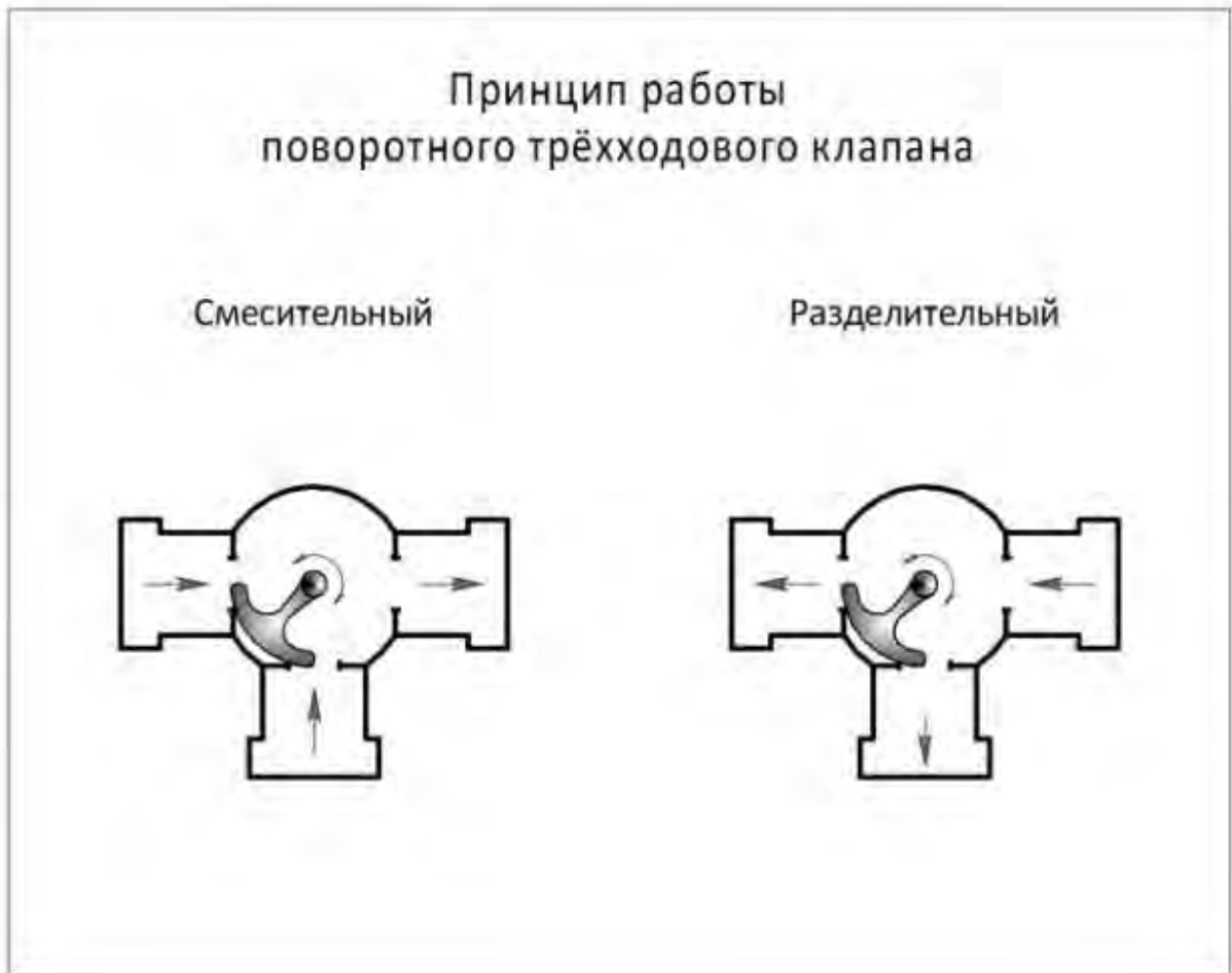
Рис. 3.7 - Трёхходовой кран
