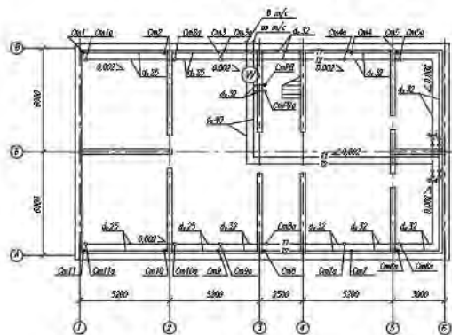
План подвала здания
