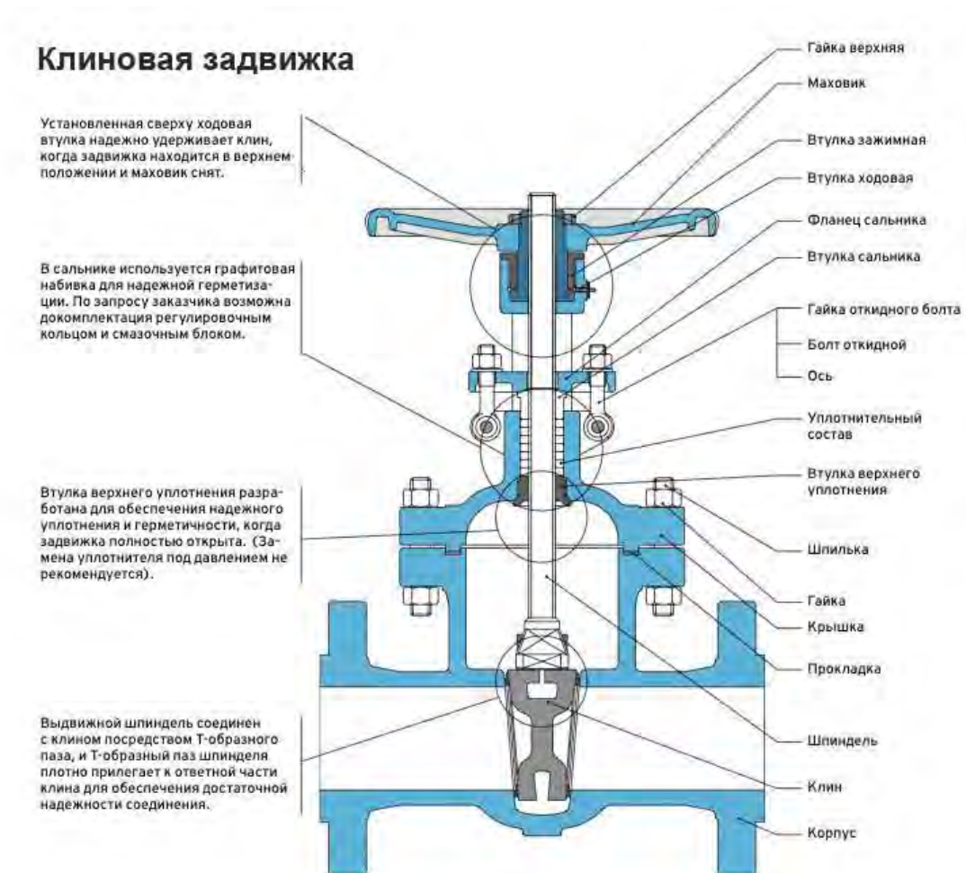
Рис. 3.5 Задвижка клиновая
