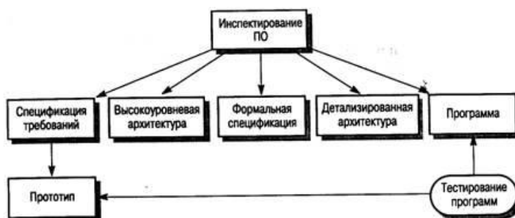
Рисунок 3. Статическая и динамическая верификация и аттестация
