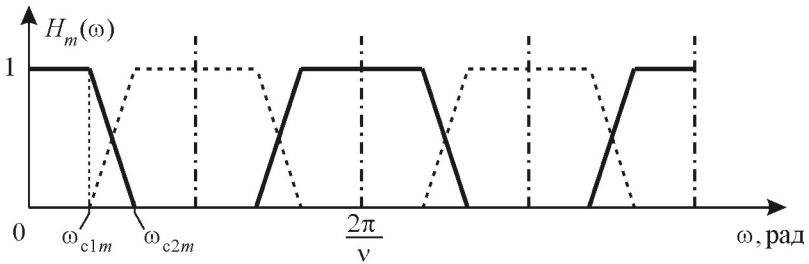
Рис. 1.4. Оптимальный многоступенчатый ЦФД: а — структурная схема; б — АЧХ фильтров
