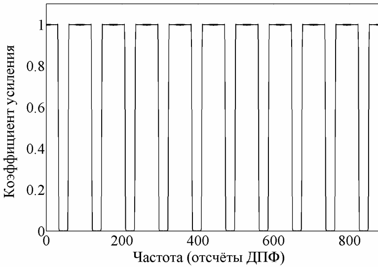
Рис. 2.4. АЧХ базового НЧ-фильтра и ЦГФ1 при \nu_{\text{опт}} = 5 и \nu_{\text{опт}} = 2 .
