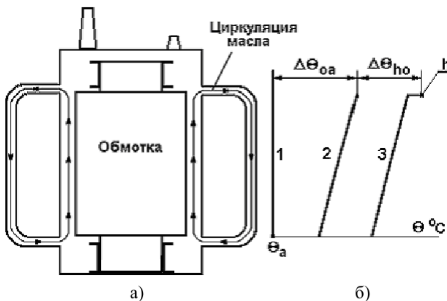
Рисунок 2 - Естественная циркуляция масла в трансформаторе (а) и тепловая диаграмма трансформатора (б)
