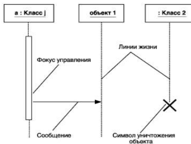
Рисунок 1 –Диаграмма последовательности
