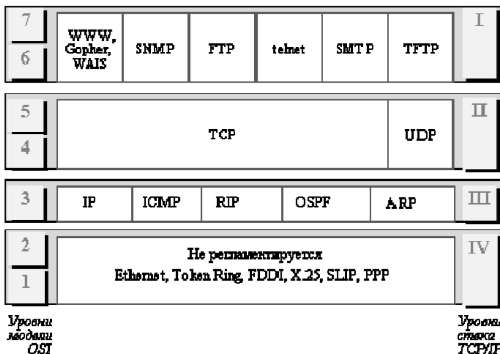
Рисунок 1 – Стек TCP/IP
