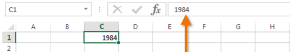
Рисунок 8 – Строка формул
