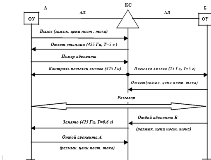
Рисунок 2 – Диаграмма обмена сигналами в процессе обслуживания абонентского телефонного вызова
