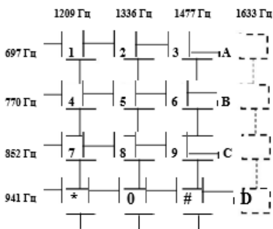
Рисунок 4 – Раскладка клавиатуры телефонного аппарата
