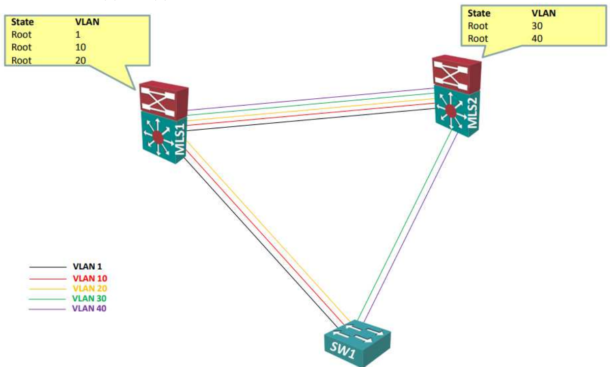
Рисунок 1 – STP- топология
