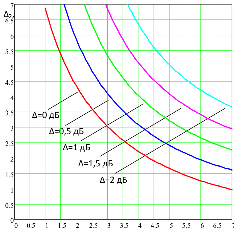
Рисунок 3.1 – Взаимная зависимость энергетического запаса на участках \Delta_1, \text{дБ}
