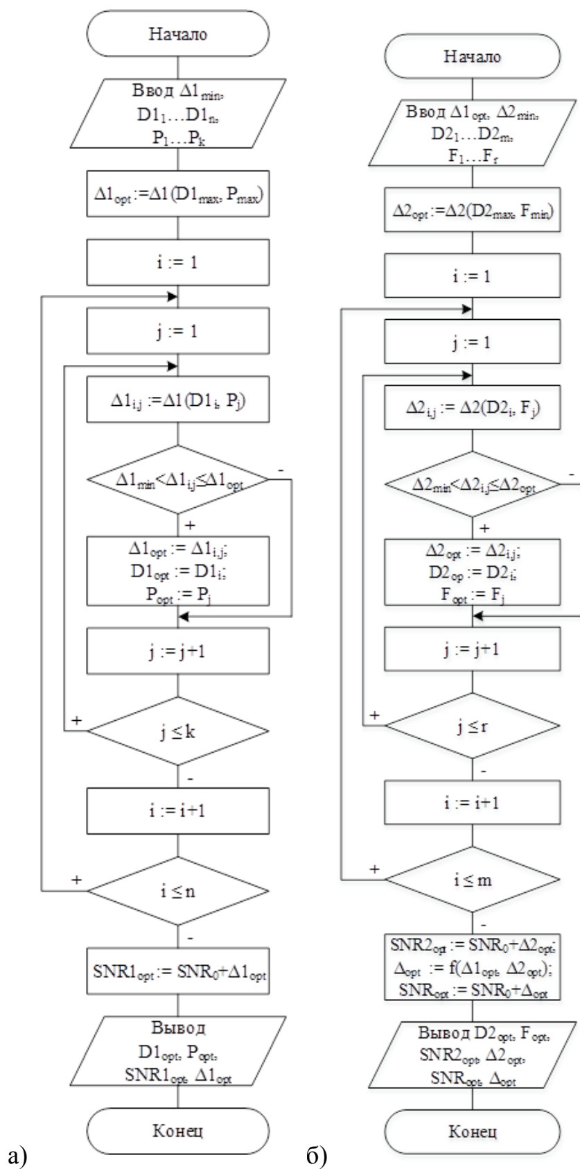
Рисунок 1 – Алгоритмы оптимизации параметров земных станций: а) ЗС 1 ; б) ЗС 2
