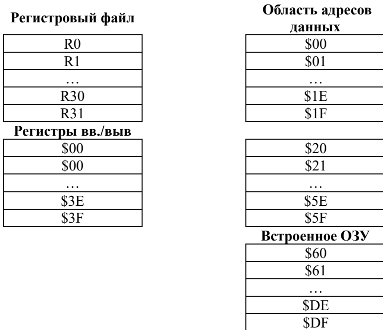
Рисунок 3- Организация памяти данных
