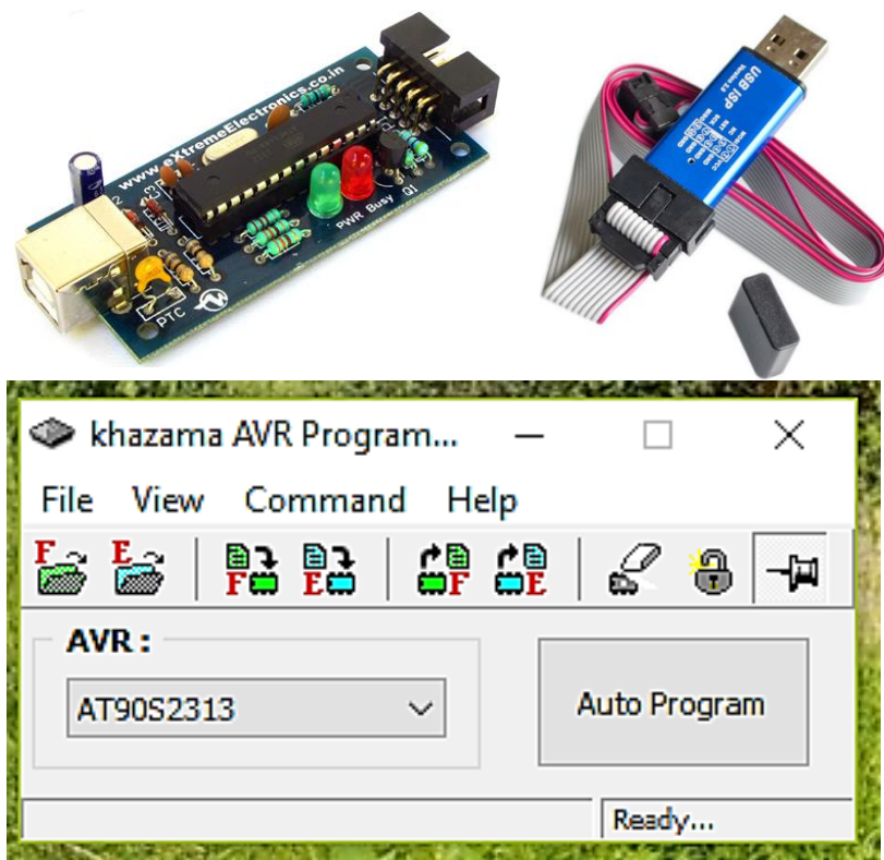
Рисунок 10 - Программатор.
