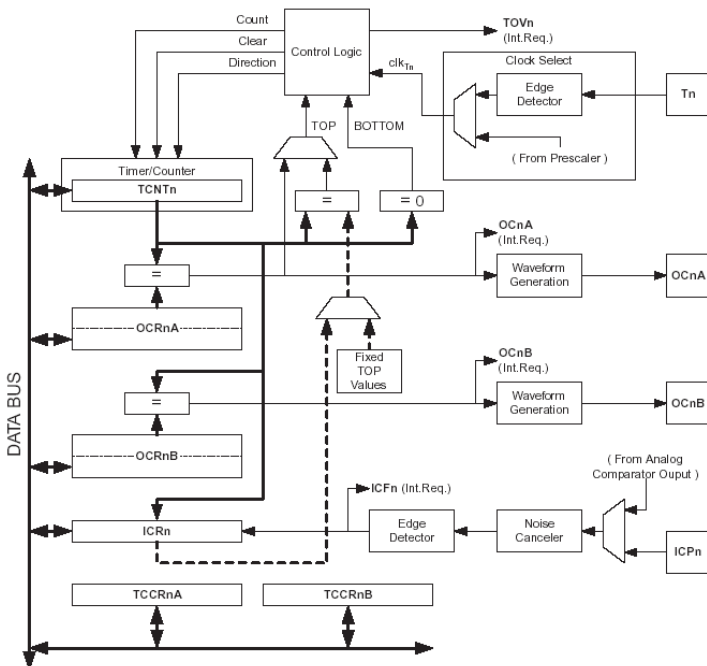
Рисунок 1 – Структурная схема таймеров
