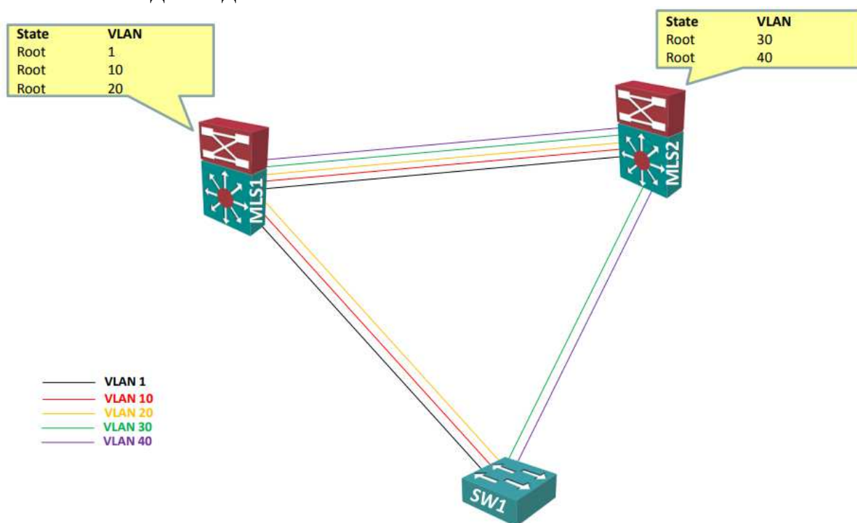
Рисунок 1 – STP- топология
