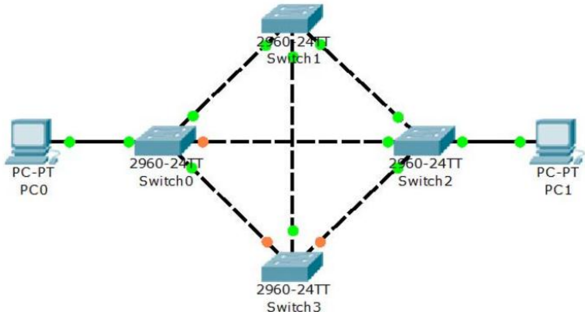
Рисунок 1 – Схема сети с избыточными линиями связи
