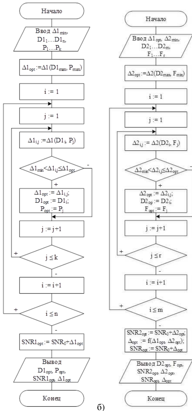
Рисунок 1 – Алгоритмы оптимизации параметров земных станций: а) 3C_1 ; б) 3C_2
