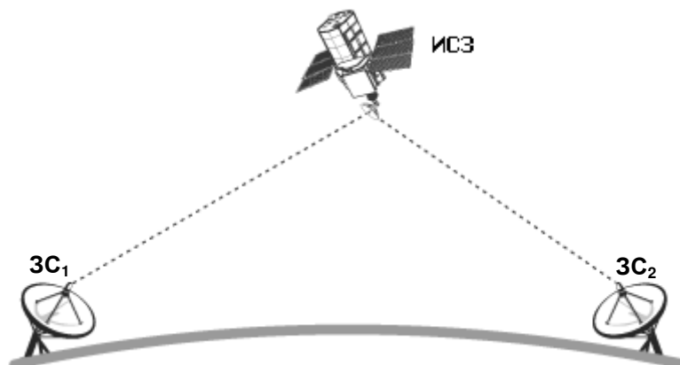
Рисунок 3 – Структурная схема спутниковой линии связи системы VSAT
