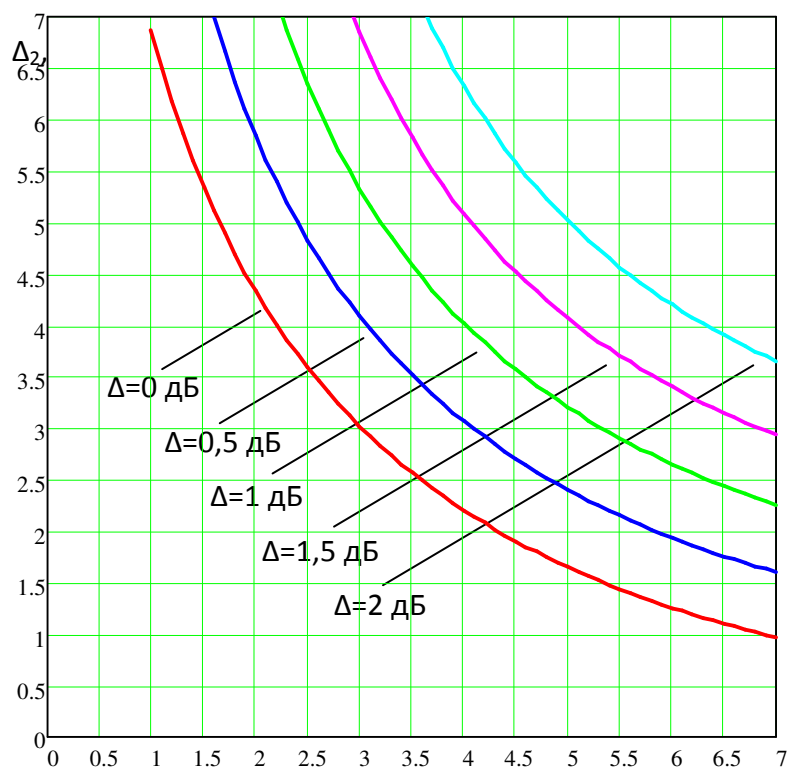
Рисунок 3.1 – Взаимная зависимость энергетического запаса на участках \Delta_1 , дБ
