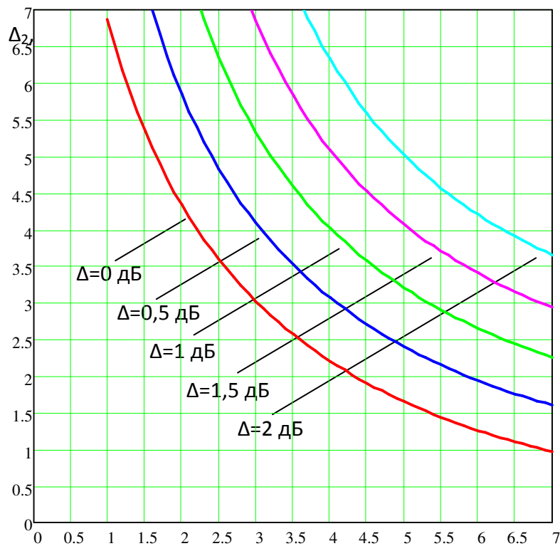
Рисунок 3.1 – Взаимная зависимость энергетического запаса на участках \Delta_1 , дБ
