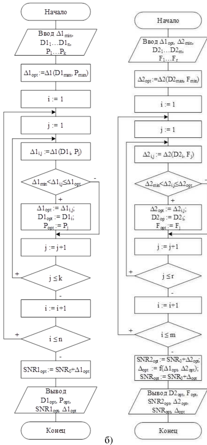
Рисунок 1 – Алгоритмы оптимизации параметров земных станций: а) ЗС 1 ; б) ЗС 2
