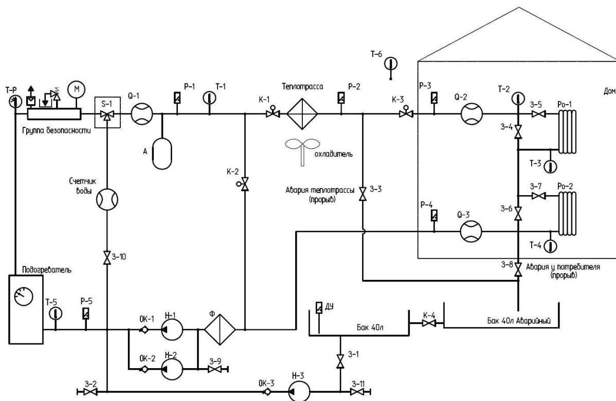
Рисунок 1– Схема гидравлическая принципиальная
