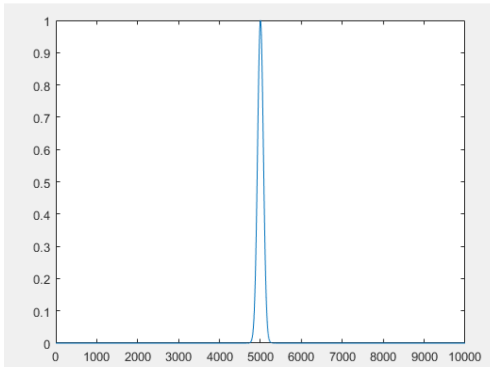
Рис. 3.4 Функция Гаусса
