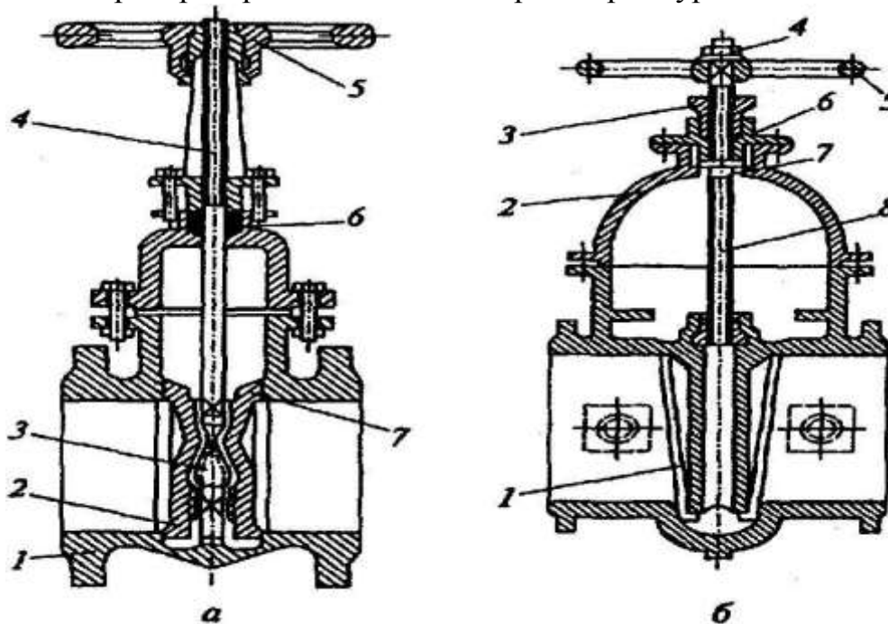
Рис. 3 – Задвижки:
