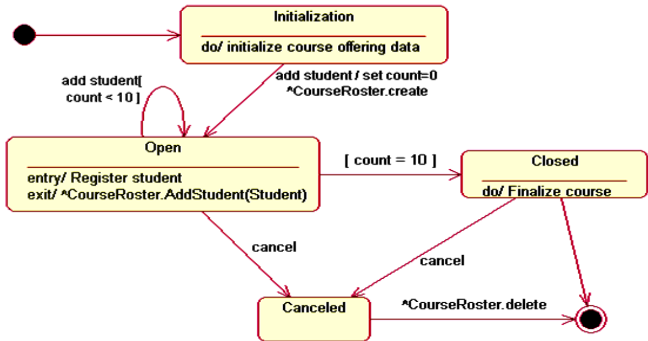
Рис. 1. Диаграмма состояний для класса CourseOffering
