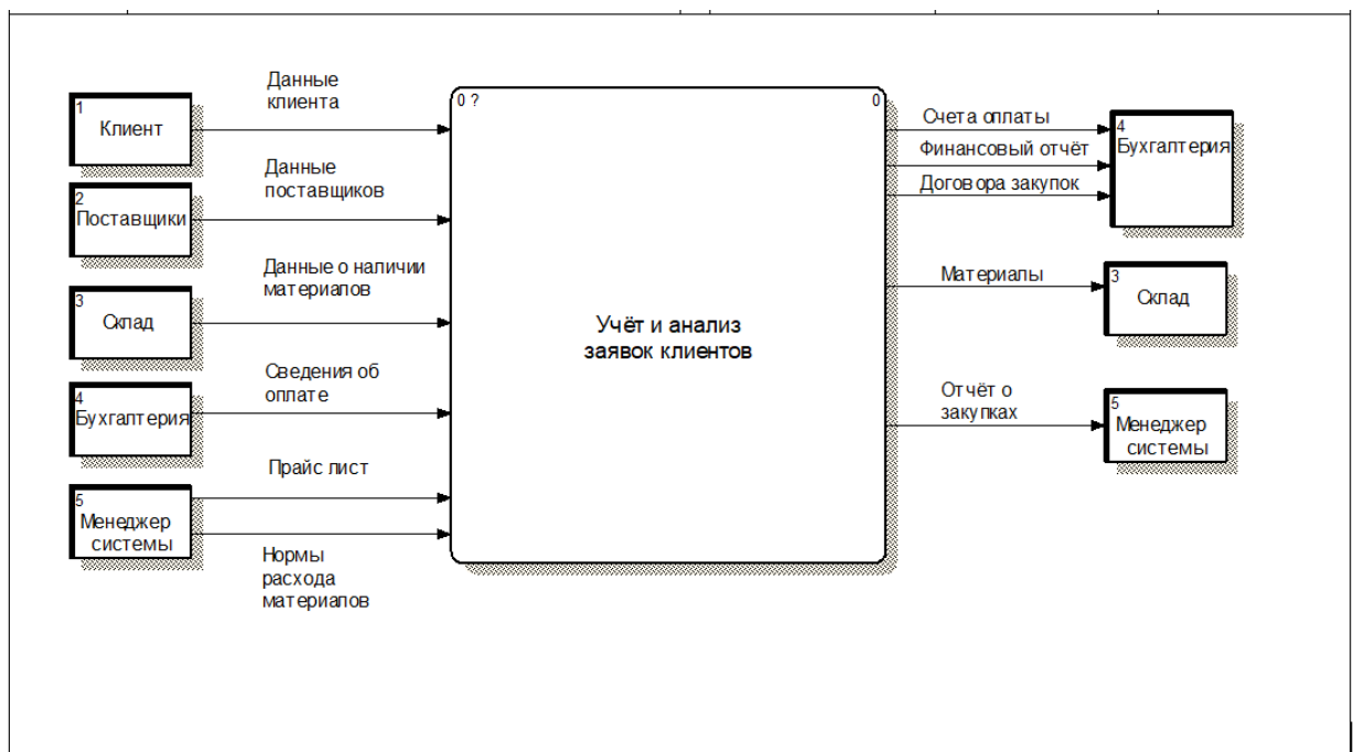
Рисунок 2 – Контекстная диаграмма в нотации DFD
