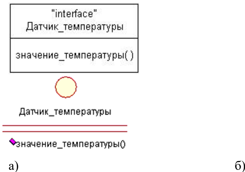
Рис. 2. Пример изображения интерфейса
