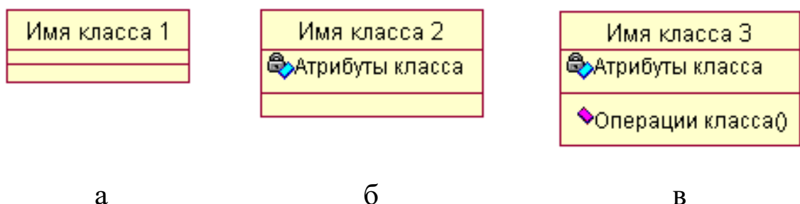
Рис. 1. Графическое изображение класса на диаграмме классов
