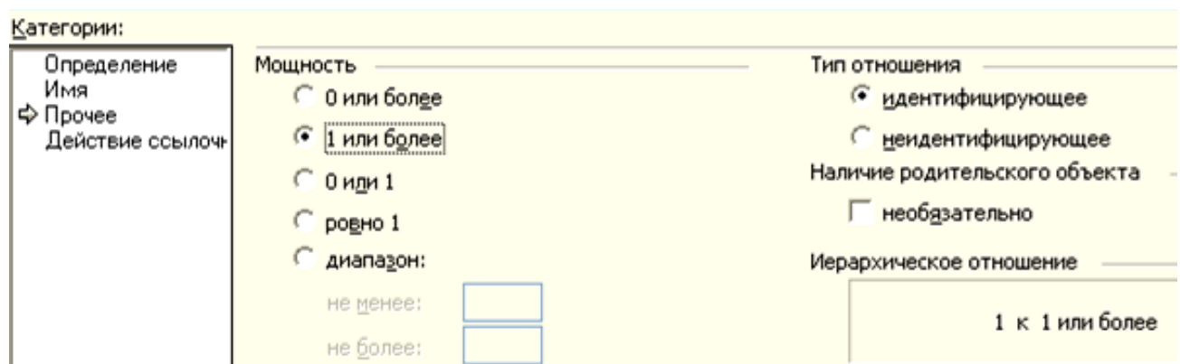
Рисунок 3 – Определение типа связи и мощности
