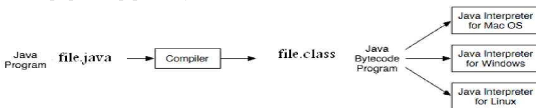
Рисунок 2.1. Создание и исполнение байт-кода
