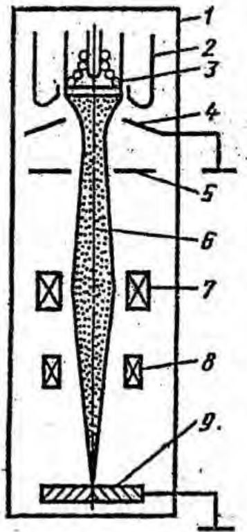
Рис. 2. Сварка электронным лучом: а – схема электронной пушки
