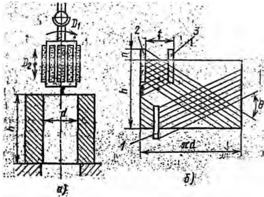
Рис. 6. Схема хонингования
