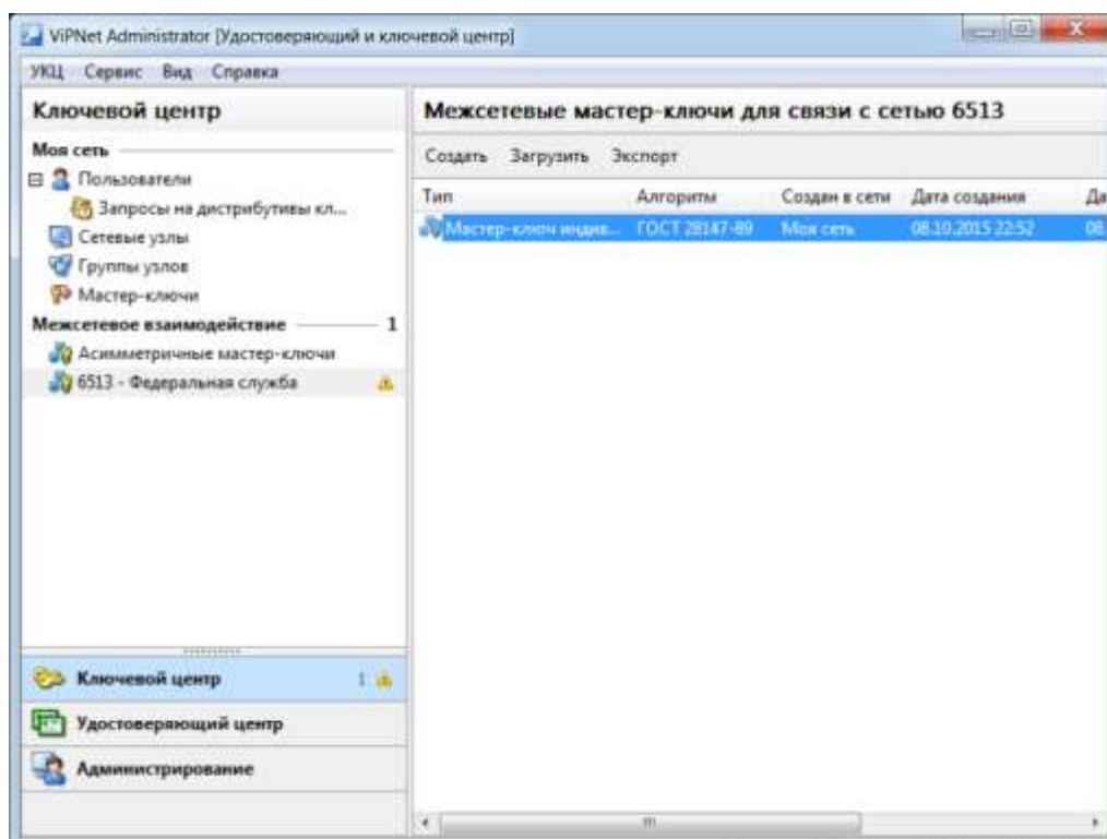
Рис. 4 – Создание ИСММК
