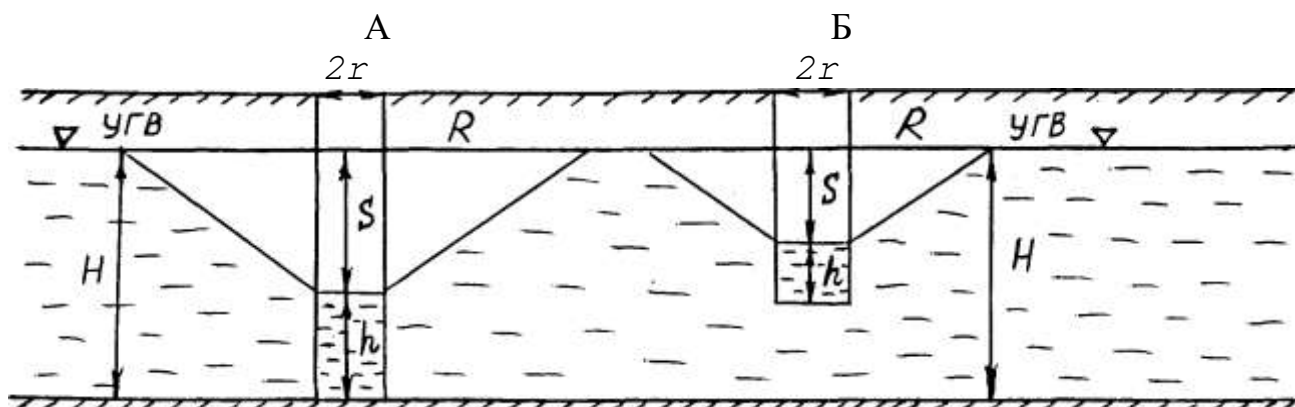
Рис. 1. Водозаборные колодцы
