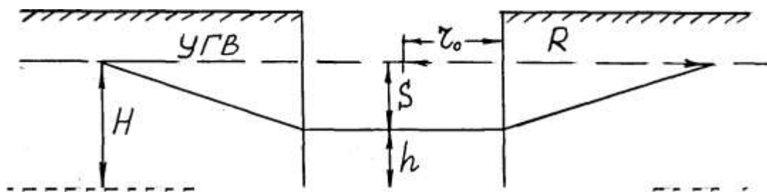
Рис. 4. Приток грунтовых вод в котлован
