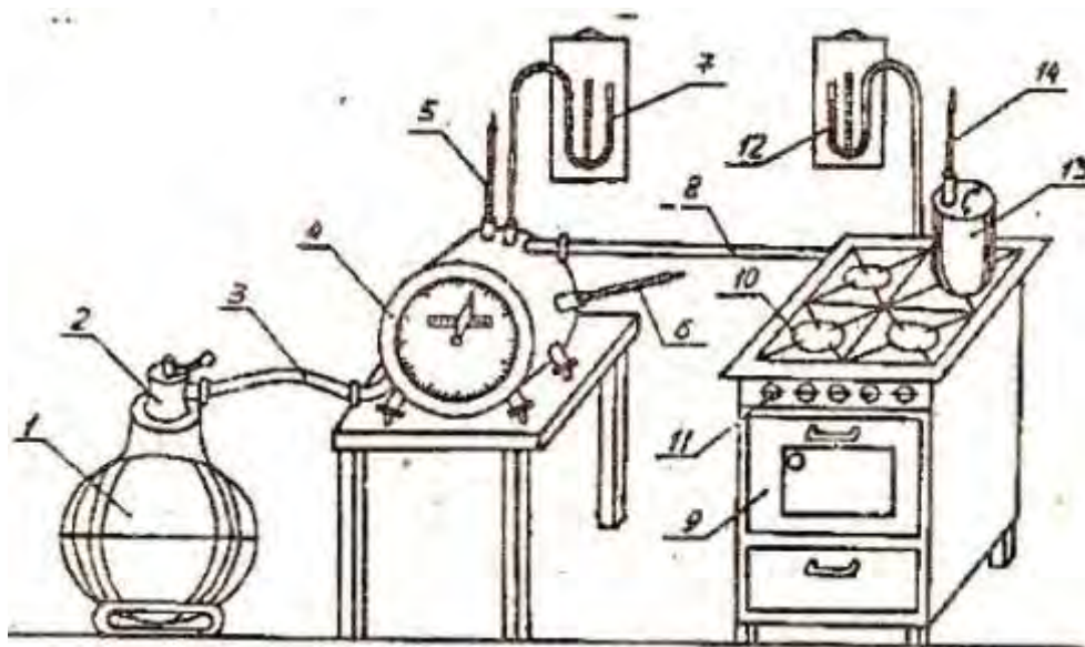
Рис. 8. Газобаллонная установка.
