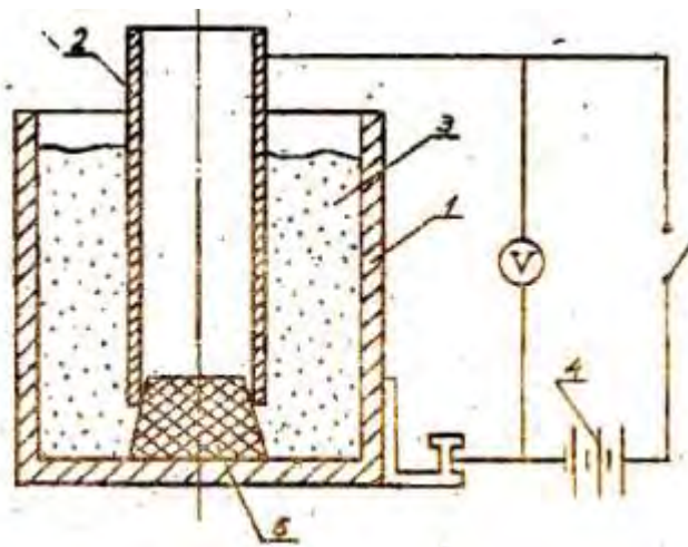
Рис 5. Устройство для определения коррозионной активности 1 - стальной сосуд; 2 - эталонный образец; 3 - исследуемый грунт; 4 - источник постоянного тока; 5 - изолирующая пробка
