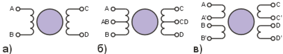
Рис. 3.4 Биполярный двигатель (а), униполярный (б) и четырехобмоточный (в)
