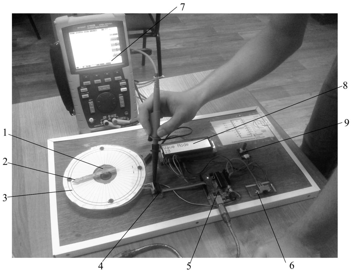
Рис. 3.6. Внешний вид стенда в процессе измерений
