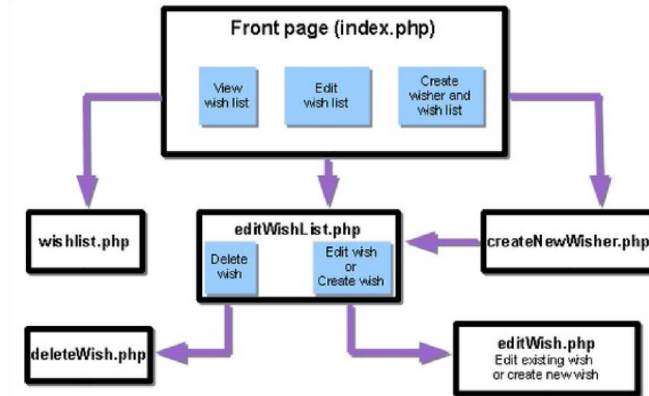
Рис. 9. Блок-схема приложения
