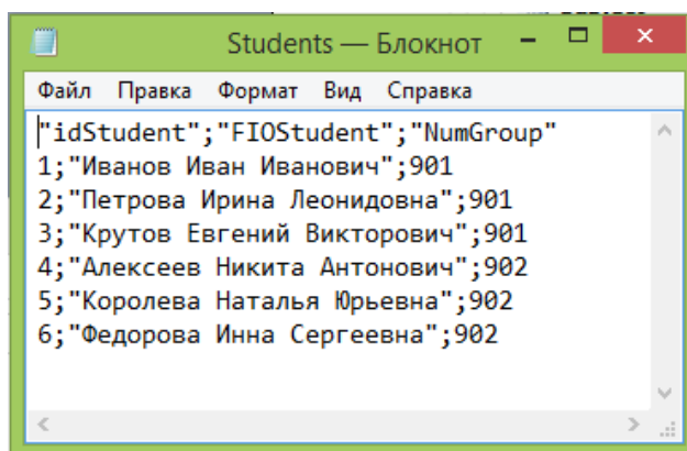
Рис. 44 - Файл «Student.csv»
