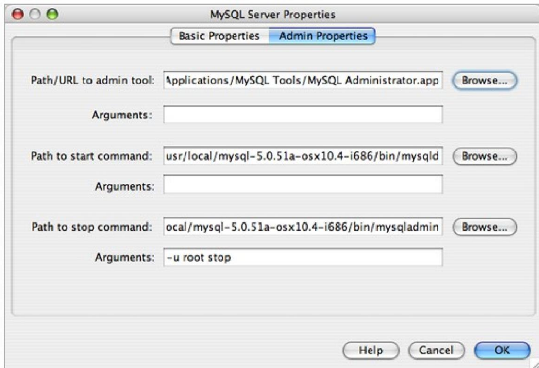
Рис. 4. Внешний вид вкладки «Свойства администратора»
