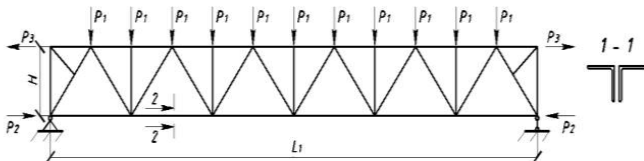
Рисунок 2.1 - Расчетная схема к лабораторной работе №3
