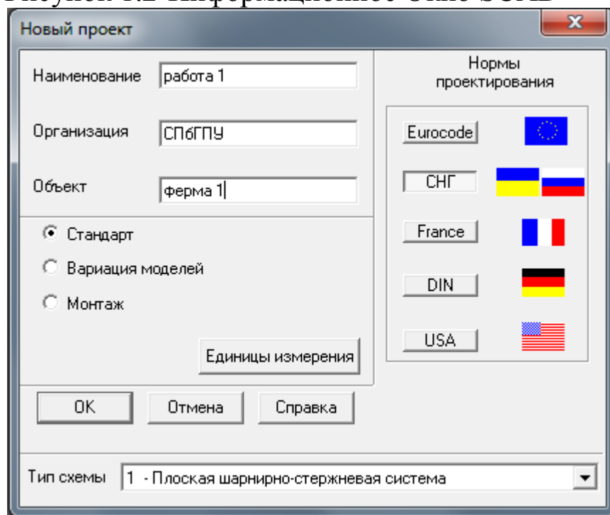
Рисунок 1.3- Диалоговое окно SCAD для создания нового проекта
