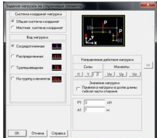
Рисунок 1.15 - Задание сосредоточенной нагрузки P_1 = 3 \text{ кН} на элемент на расстоянии a_1 = 1 \text{ м} от левого его края вдоль оси Z
