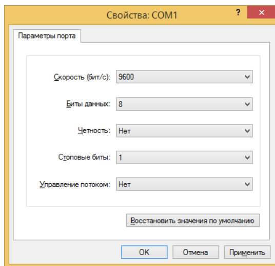
Рисунок 3 – Вводим стандартные характеристики консольного порта
