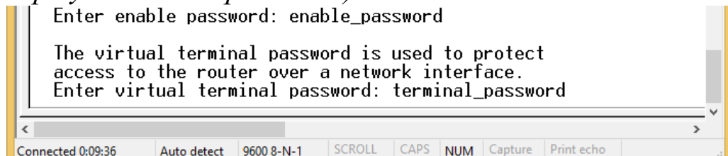
Рисунок 9 – Ввод пароля виртуального терминала
