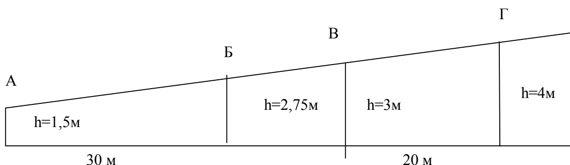
Рисунок 1 - Продольный разрез траншеи
