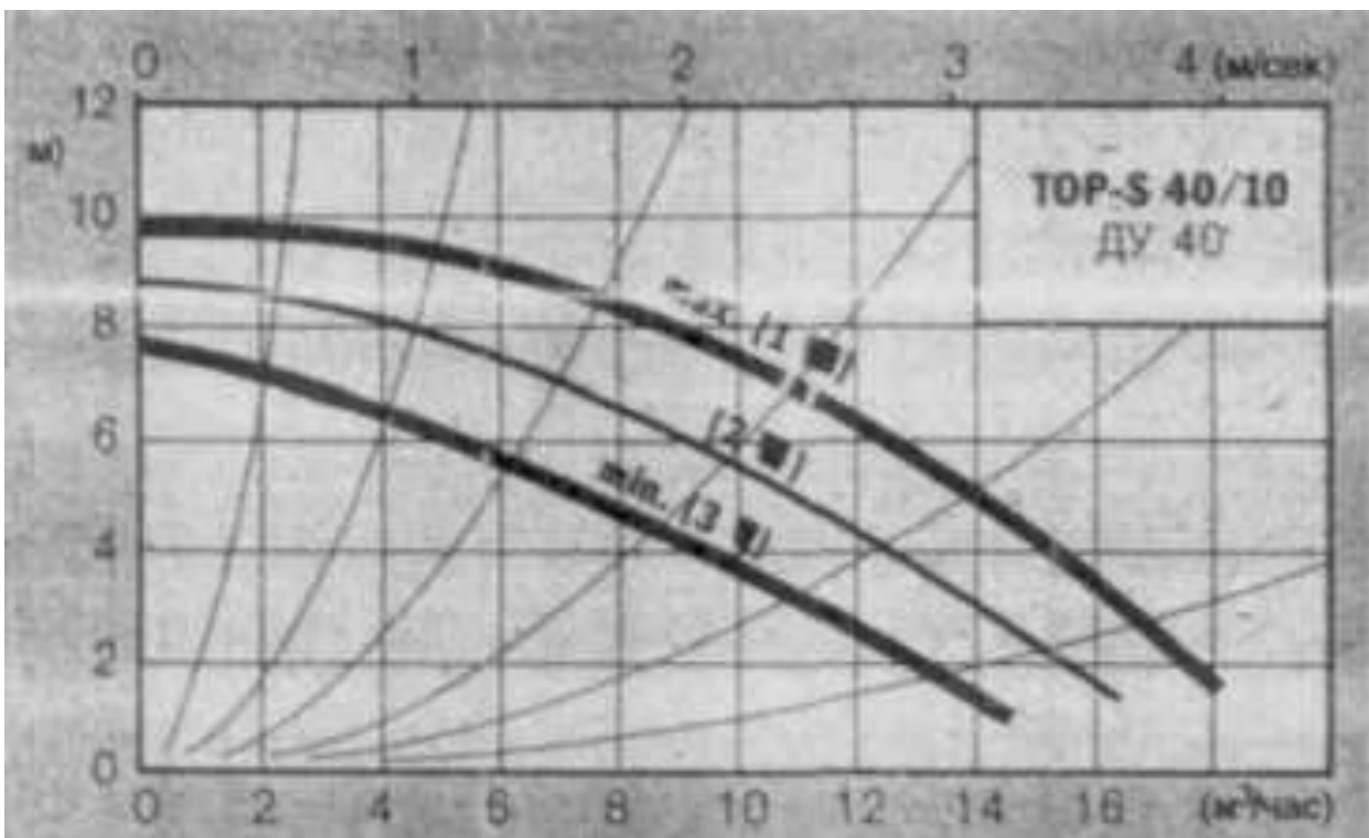
Рис.П.6.8. Характеристики регулируемых электронасосов типоряда TOP-S ( n = 2800 об/мин, крутая характеристика)
