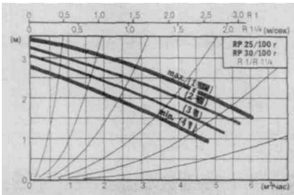
Рис.П.6.12. Характеристики регулируемых электронасосов типа RP-S ( n = 1400 об/мин, пологая характеристика)
