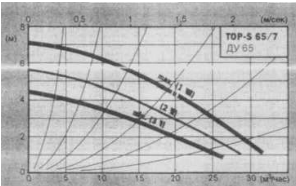
Рис.П.6.10. Характеристики регулируемых электронасосов типоряда TOP-S ( n = 2800 об/мин, крутая характеристика)
