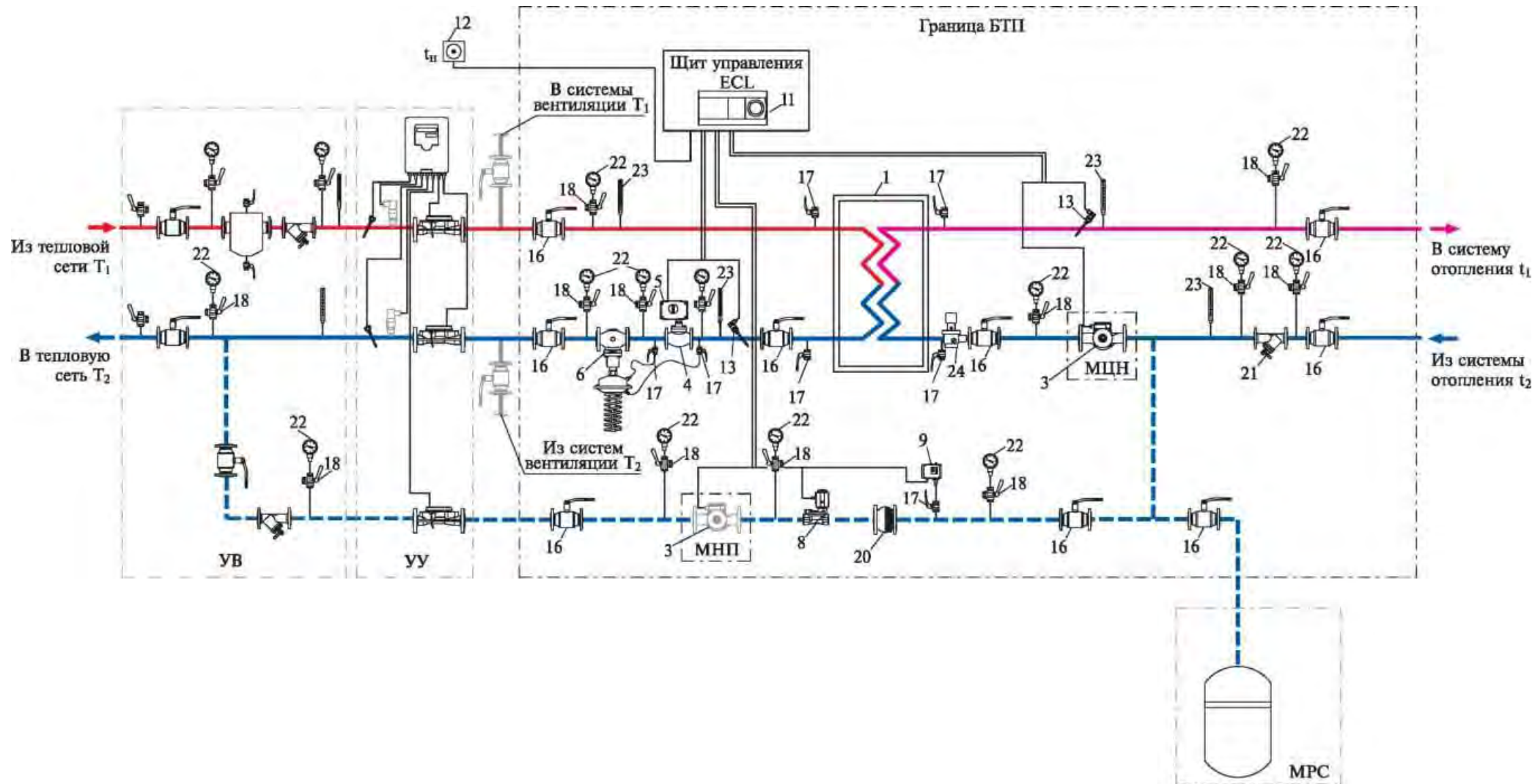
Рис.1. Схема АИТП при независимом присоединении системы отопления к тепловой сети (обозначение позиций см. прилож.2.)
