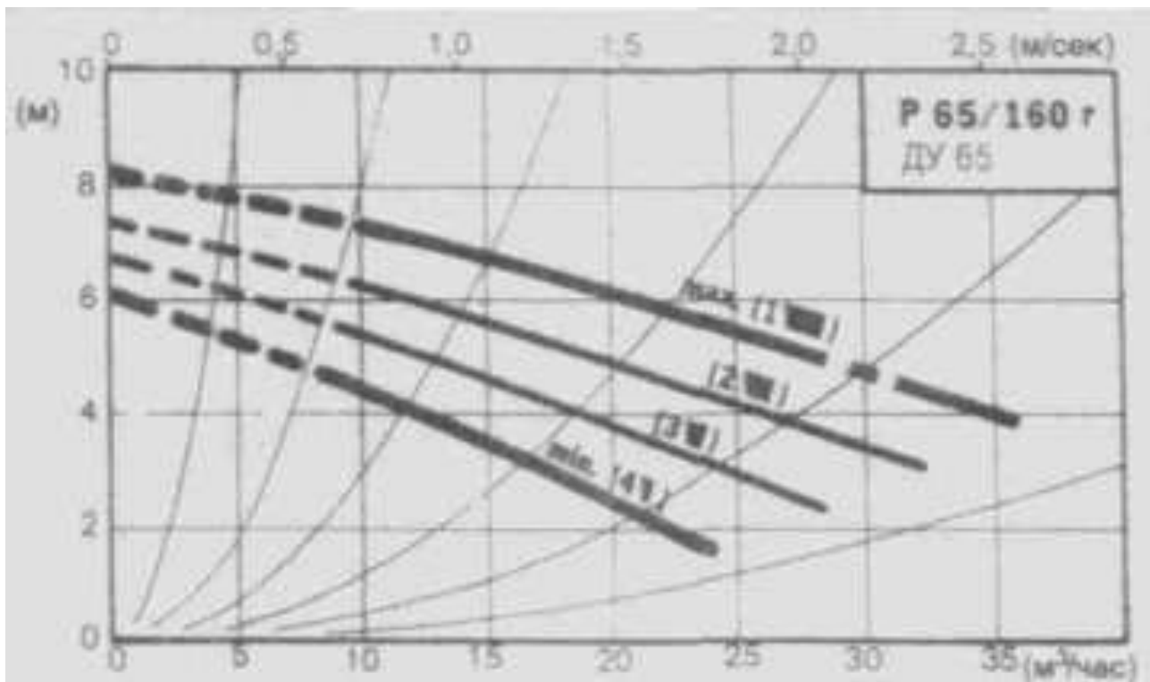
Рис.П.6.15. Характеристики регулируемых электронасосов типорядаР ( n = 1400 об/мин, пологая характеристика)
