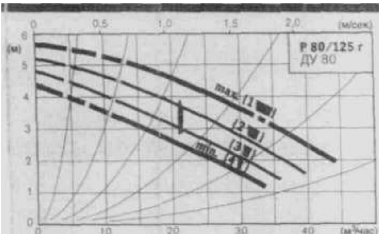
Рис.П.6.17. Характеристики регулируемых электронасосов типорядаР ( n = 1400 об/мин, пологая характеристика)
