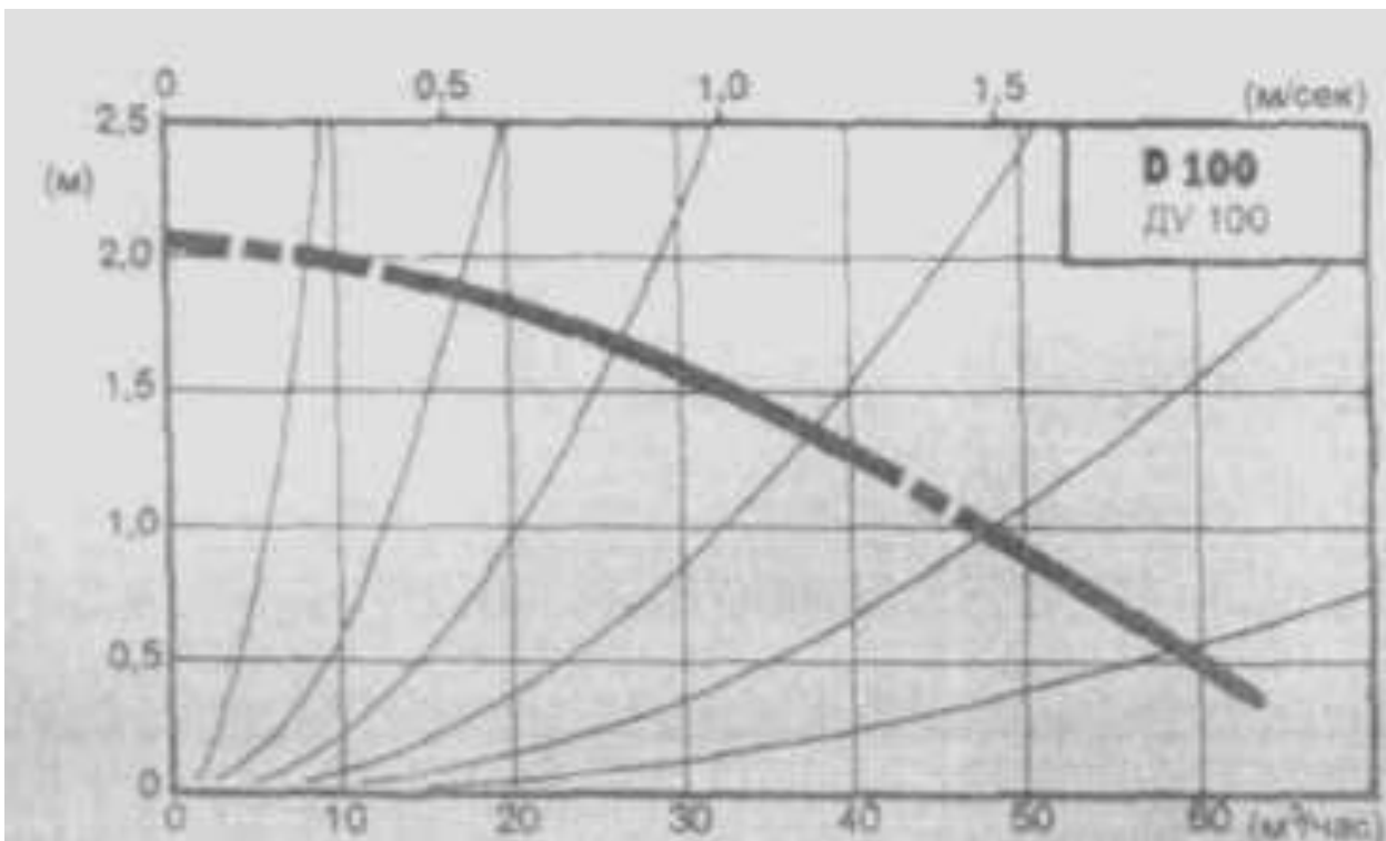
Рис.П.6.21. Характеристики регулируемых электронасосов типа D (n = 1400 об/мин, пологая характеристика)
