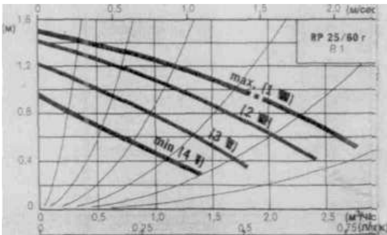
Рис.П.6.11. Характеристики регулируемых электронасосов типоряда TOP-S ( n = 2800 об/мин, крутая характеристика) и типоряда RP-S ( n = 1400 об/мин, пологая характеристика)
