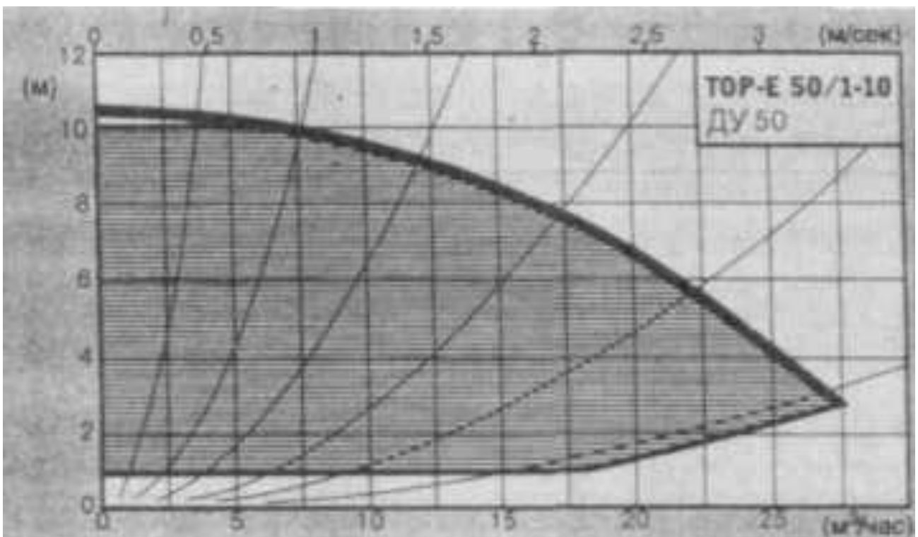
Рис.П.6.1. Характеристики регулируемых электронасосов типа TOR-E ( n – бесступенчатое)
