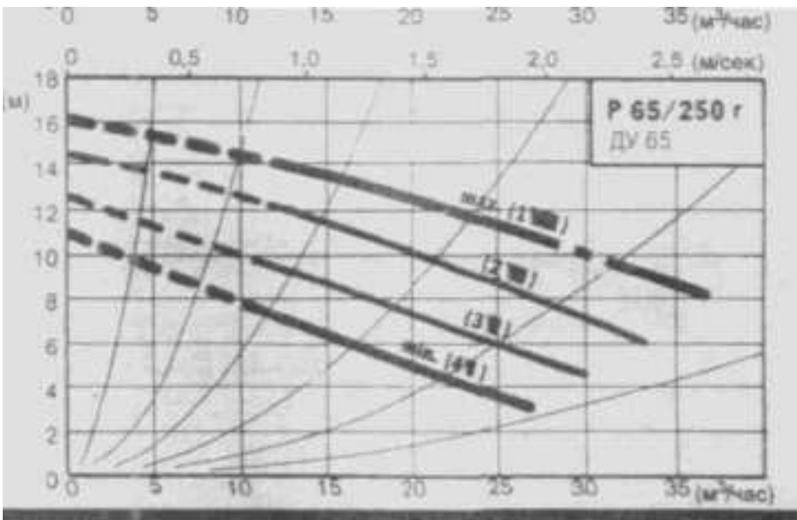
Рис.П.6.16. Характеристики регулируемых электронасосов типорядаР ( n = 1400 об/мин, пологая характеристика)
