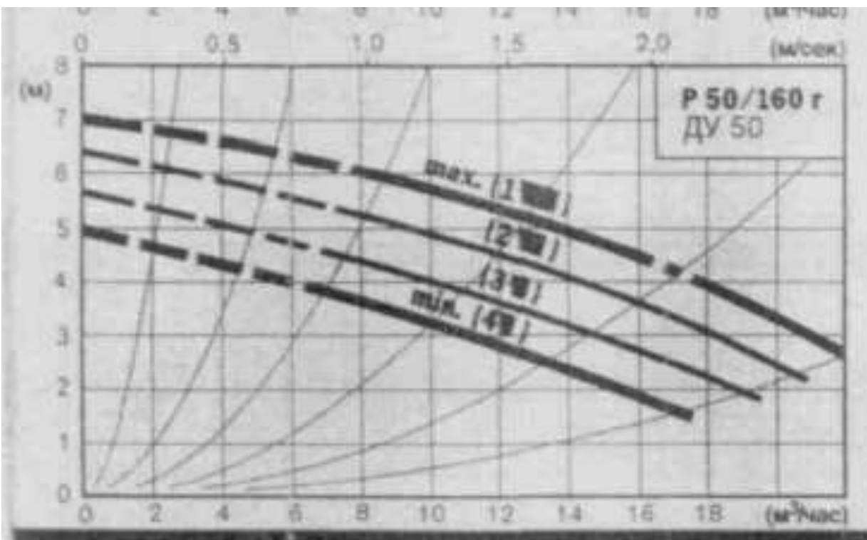
Рис.П.6.14. Характеристики регулируемых электронасосов типорядаР ( n = 1400 об/мин, пологая характеристика)
