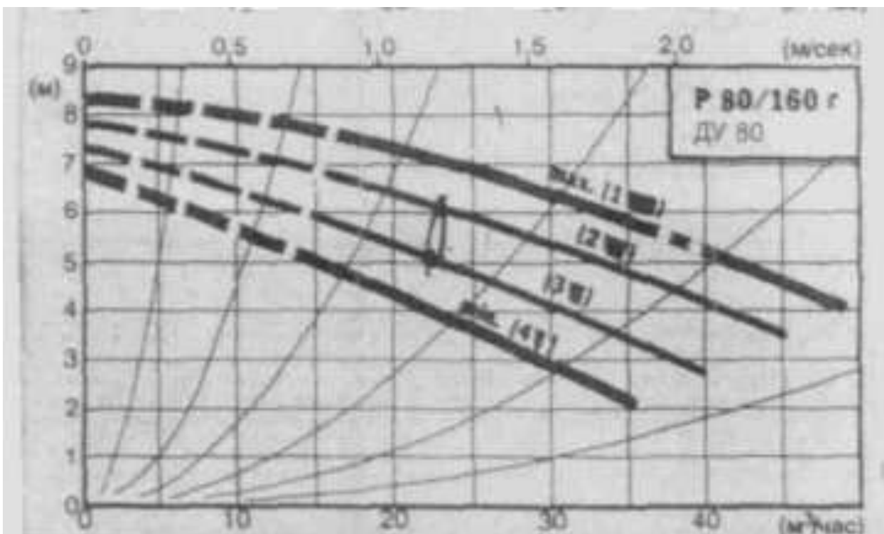
Рис.П.6.18. Характеристики регулируемых электронасосов типорядаР ( n = 1400 об/мин , пологая характеристика)
