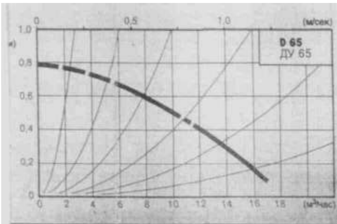
Рис.П.6.20. Характеристики регулируемых электронасосов типорядаD ( n = 1400 об/мин , пологая характеристика)
