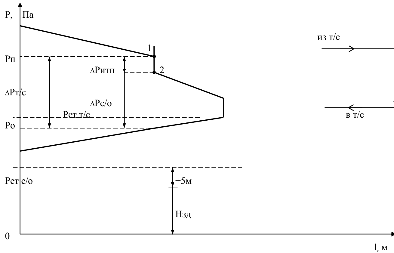
Рис. 4. Пьезометрический график при АУУ с элеваторным смещением
