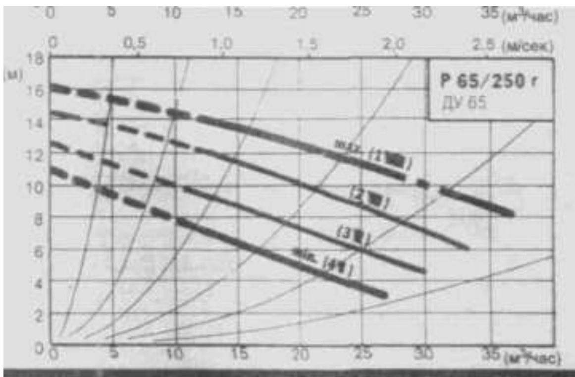
Рис.П.6.16. Характеристики регулируемых электронасосов типорядаР ( n = 1400 об/мин , пологая характеристика)
