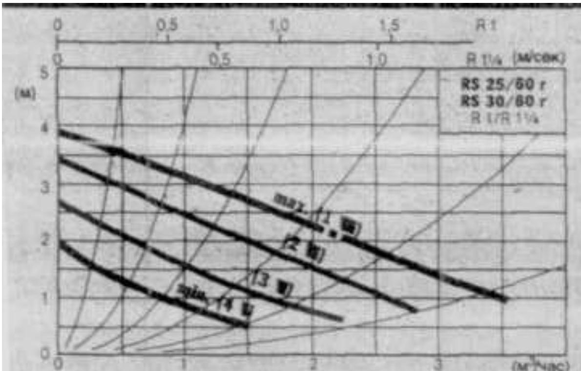
Рис.П.6.5. Характеристики регулируемых электронасосов типа RS ( n = 2800 об/мин, крутая характеристика )
