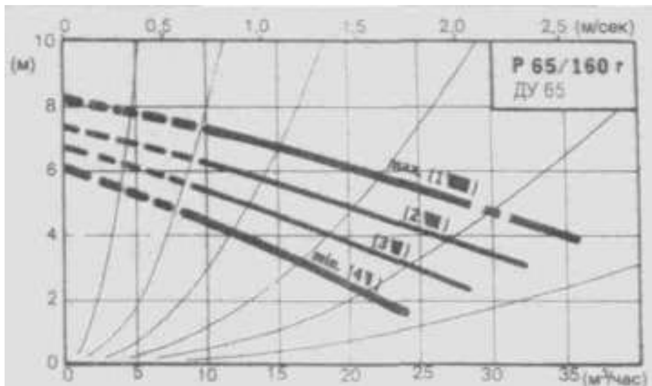
Рис.П.6.15. Характеристики регулируемых электронасосов типоряда P ( n = 1400 об/мин, пологая характеристика)
