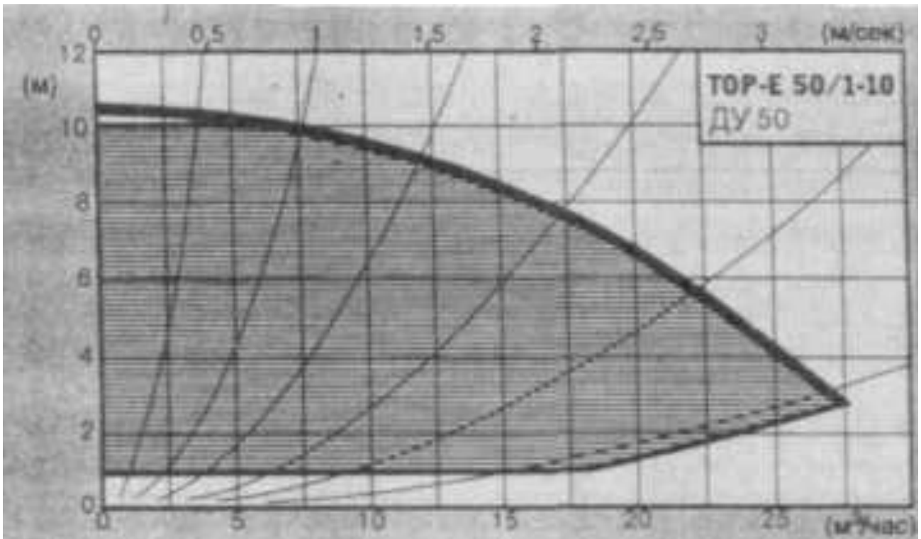
Рис.П.6.1. Характеристики регулируемых электронасосов типорядаТОР-Е (n – бесступенчатое)
