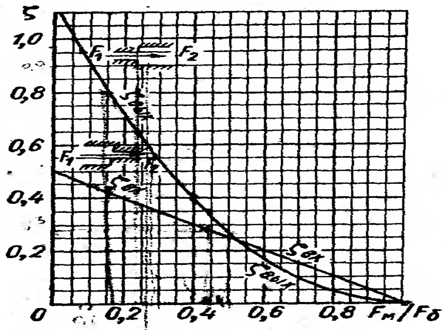
Рисунок П 1.8 - Коэффициент сопротивления при внезапном изменении сечения каналов ( F_m F_\delta – меньшее и большее сечение каналов)
