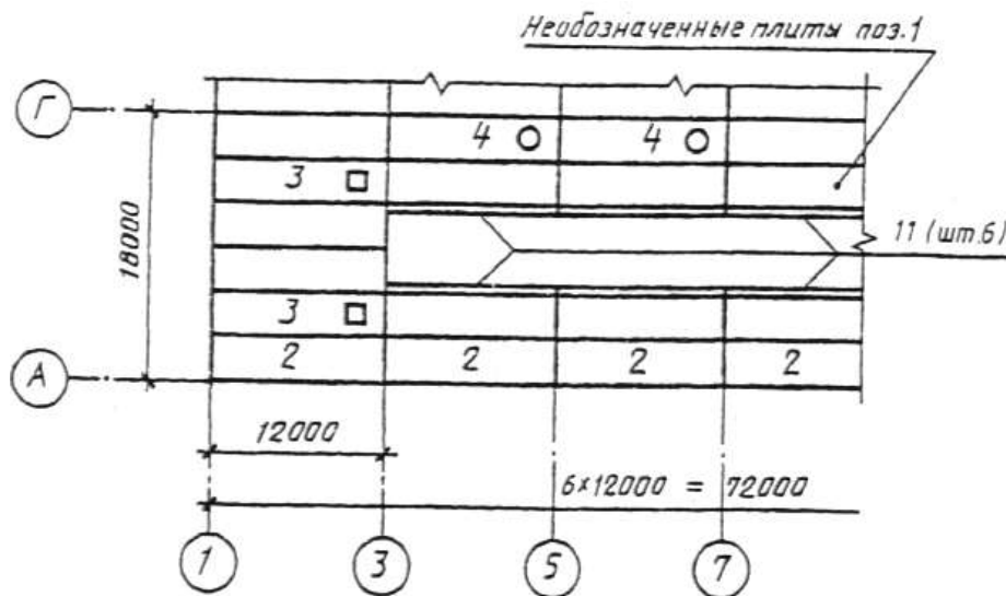
Рисунок 5 – Схема расположения плит покрытия
