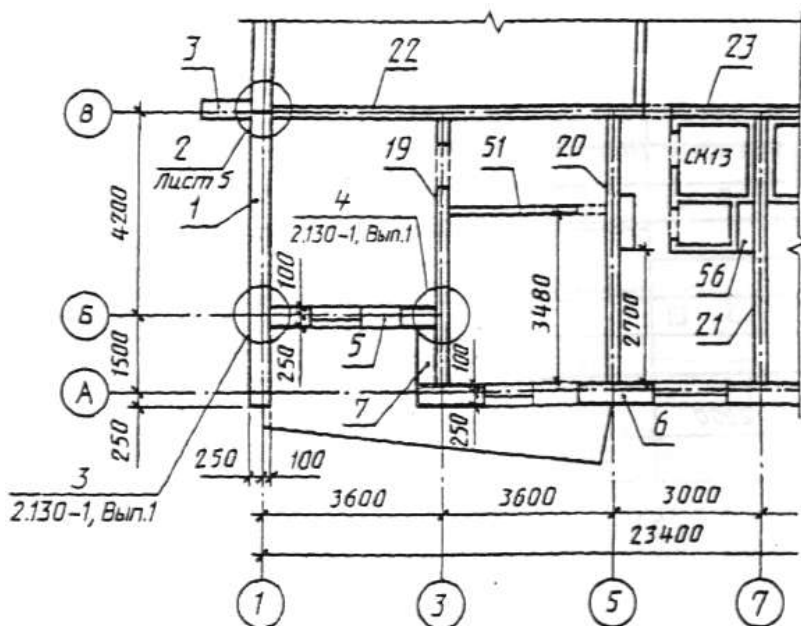
Рисунок 6 – Схема расположения панелей стен и перегородок
