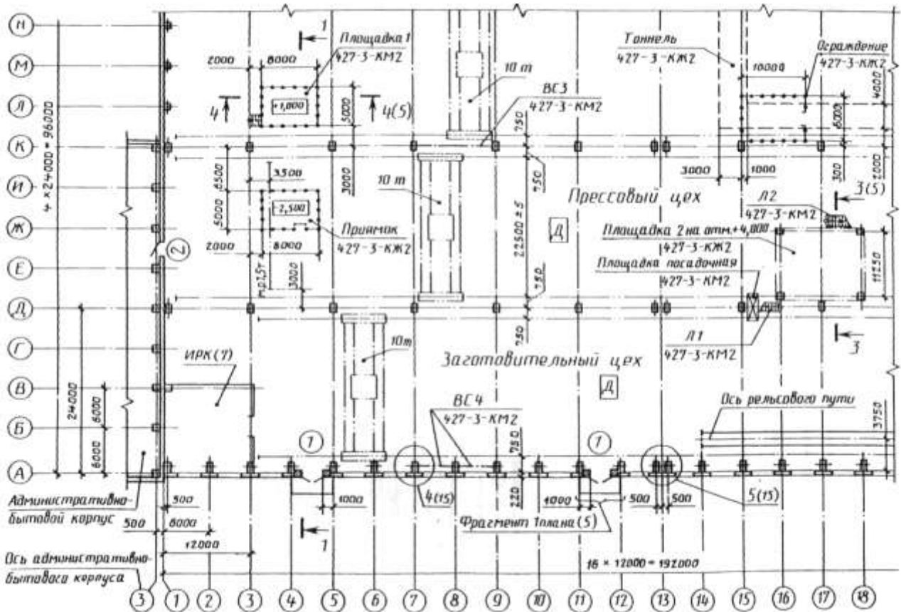
Рисунок 2 - Пример выполнения плана этажа жилого дома
