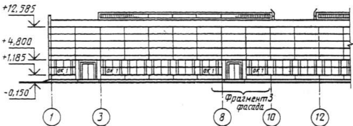
Рисунок 4 - Пример выполнения фасада жилого дома
