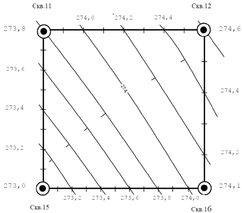
Рис 1. План расположения скважин с абсолютными отметками уровня воды.
