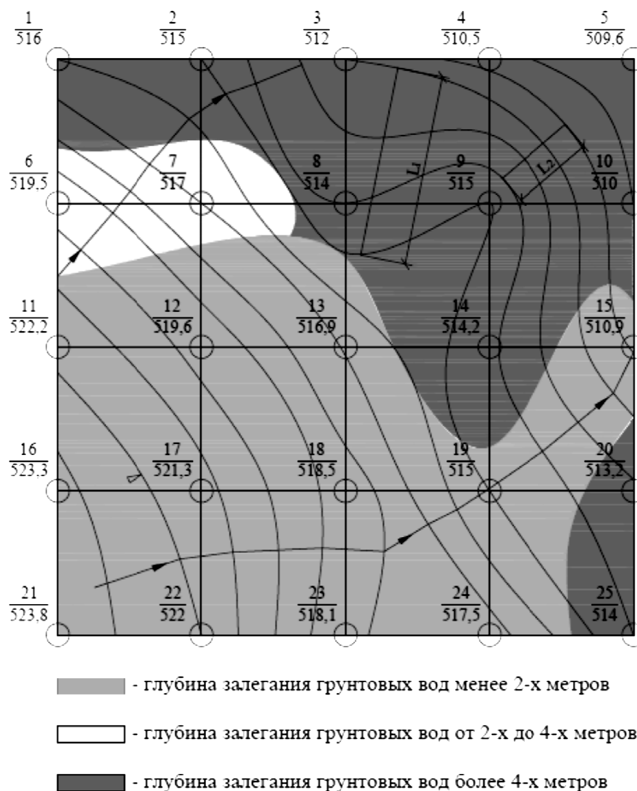
Рис 2. Построение гидроизогипс методом интерполяции в квадрате, опирающемся на четыре ближайшие скважины
