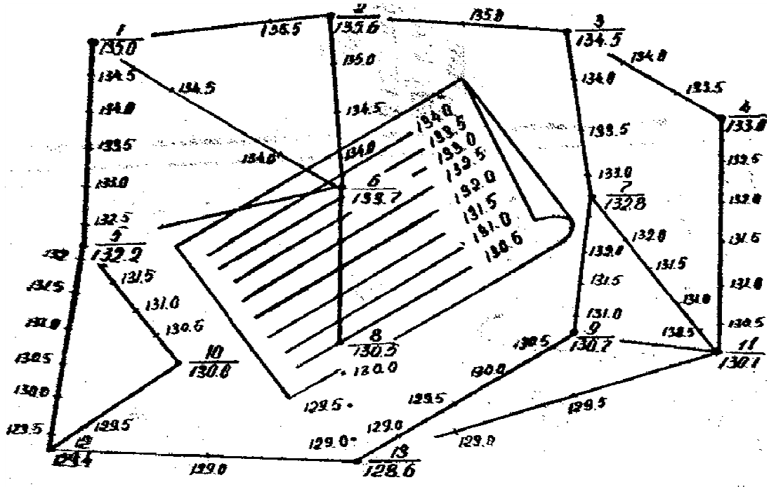
Рис 1. План расположения скважин с абсолютными отметками уровня воды.
