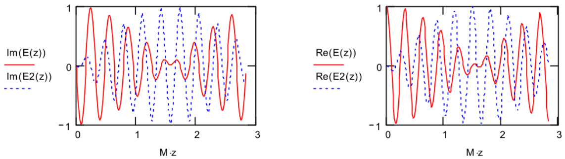
Рисунок 6 – Напряжённости мод в первом и втором волноводах
