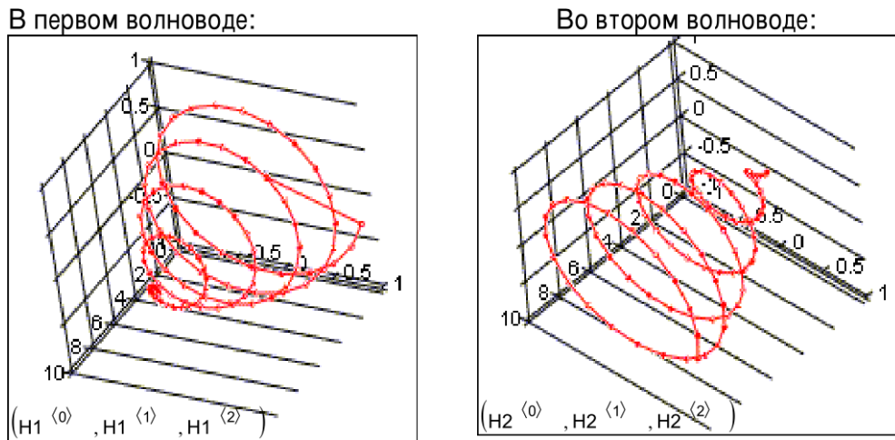
Рисунок 7 – Трёхмерное представление напряжённостей мод в волноводах
