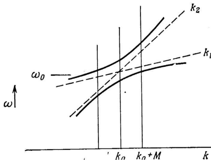
Рисунок 4 – График зависимости \omega от k для двух мод в отсутствие связи.
