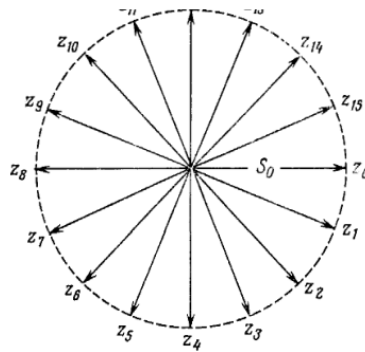
Рисунок 2 – Поляризация векторов
