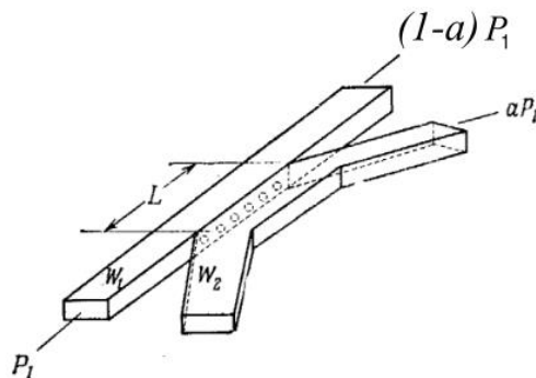
Рисунок 1 – Направленный ответвитель
