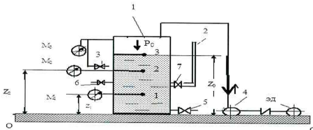
Рис.2 Схема стенда
