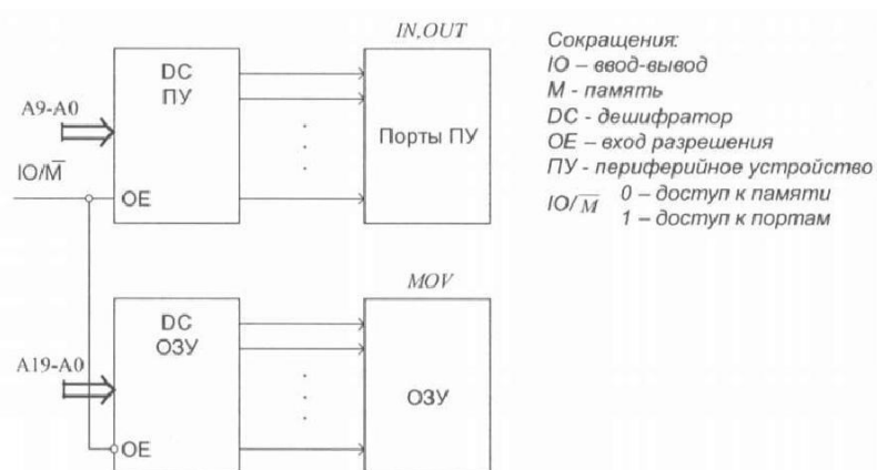
Рис. 5 – Разделенные адресные пространства ПУ и ОЗУ
