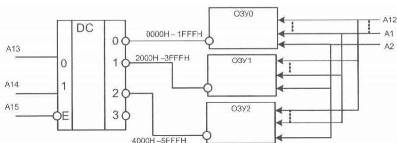
Рис. 7 - Схема дешифрации адресов
