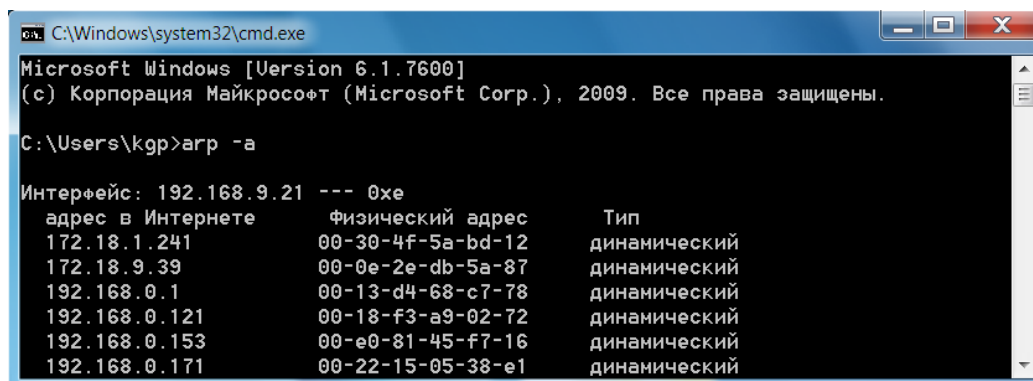
Рис. 4. Пример ARP-таблицы
