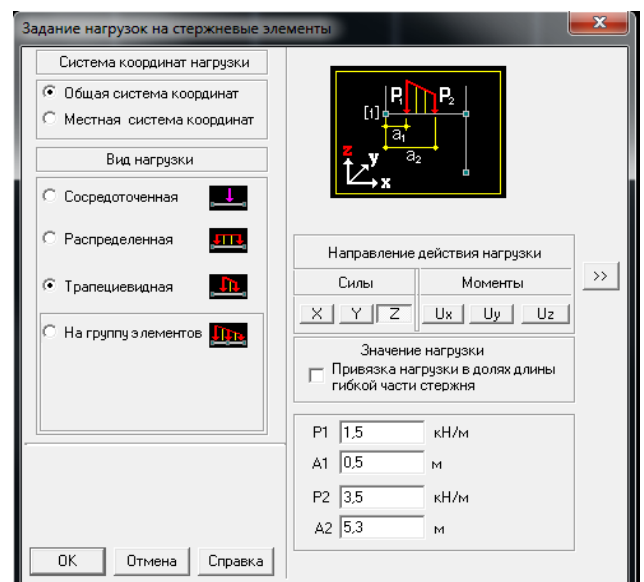
Рисунок 1.17 - Задание трапециевидной нагрузки на элемент q_2 = 1,5 \text{ кН/м} ; q_3 = 3,5 \text{ кН/м} ; a_2 = 0,5 \text{ м} ; a_3 = 5,3 \text{ м}
