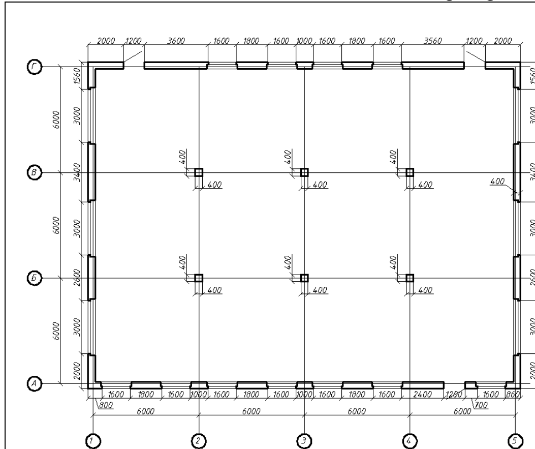
Рисунок – план типового этажа для выполнения лабораторной работы №4. Вариант 1
