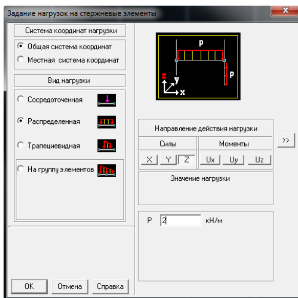
Рисунок 1.16 - Задание равномерно распределенной нагрузки на элемент q_1 = 2 \text{ кН/м}
