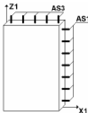
Рисунок 4.22 - Балка-стенка
