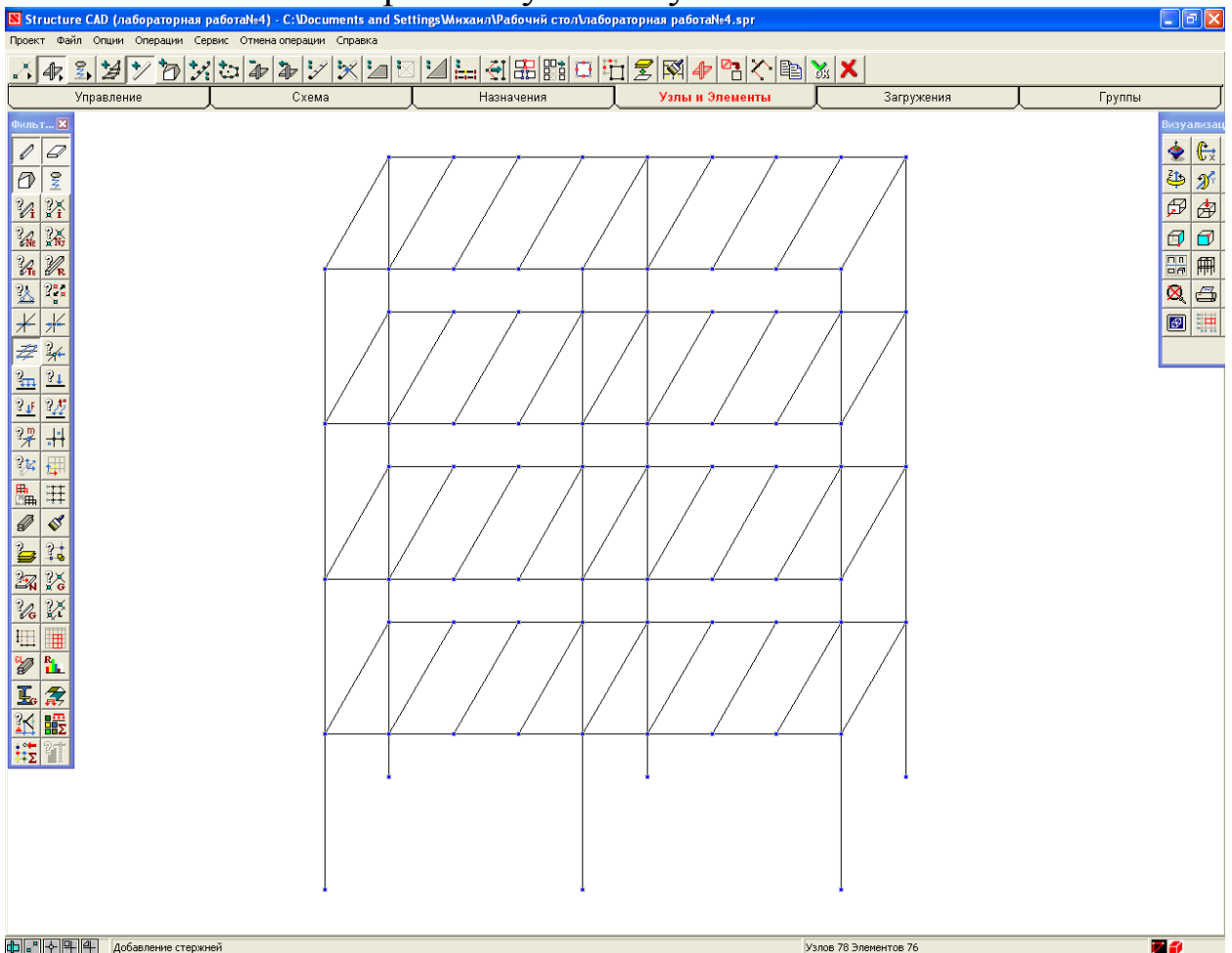
Рисунок 3.12 – Модель пространственной рамы
