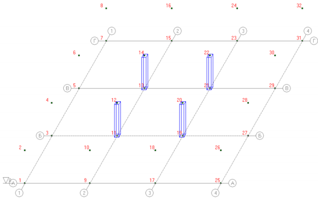
Рисунок 4.11 – Схема с колоннами в подпроцессоре Форум
