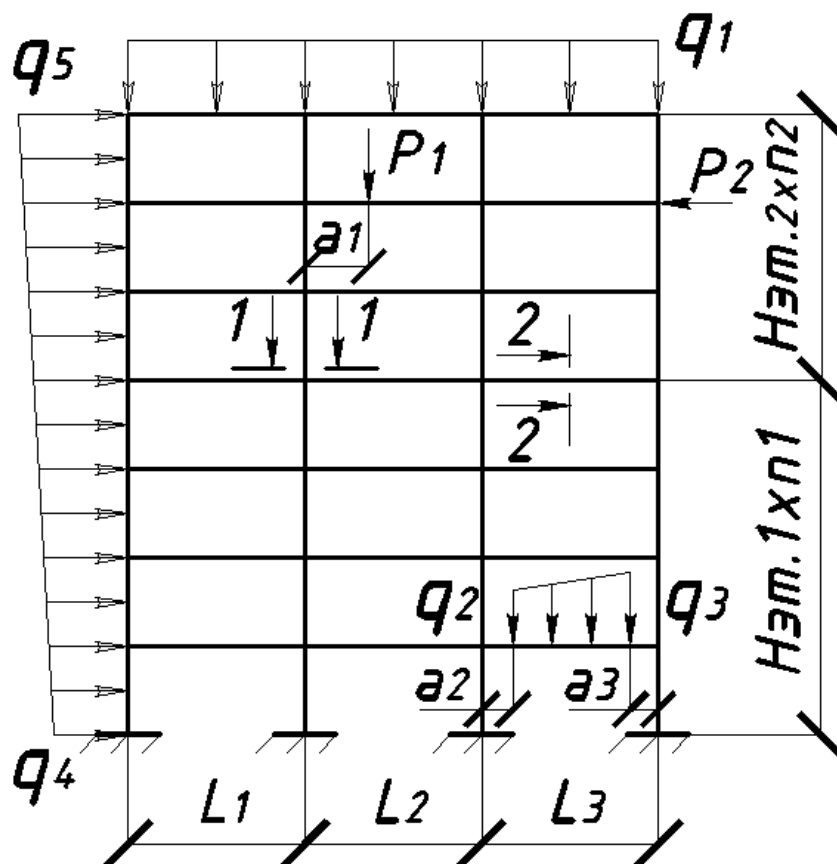
Рисунок 1.1 — Расчетная схема к лабораторной работе №1
