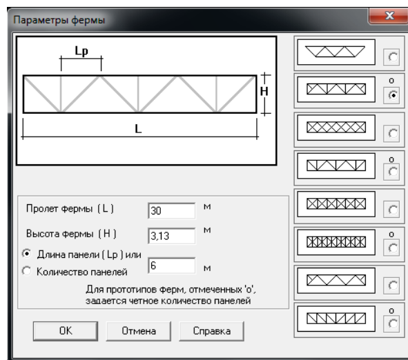
Рисунок 2.9 - Выбор варианта решетки и задание параметров фермы: пролет L=30 м, высота фермы H=3,13 м, длина панели L_p=6 м.
