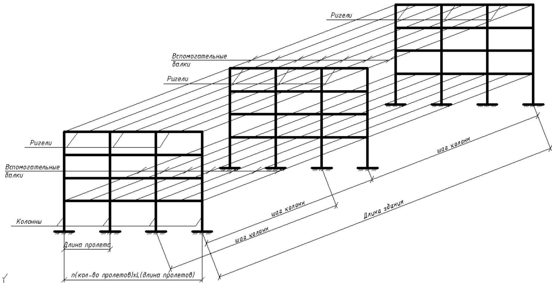
Рисунок 2.1 – Расчетная схема к лабораторной работе №2 (вспомогательные балки 2-го и 3-го этажей условно не показаны)
