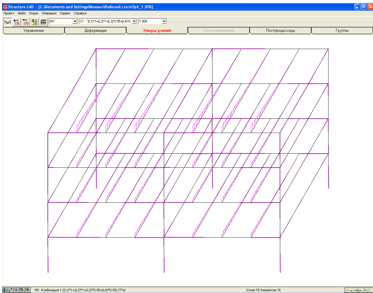
Рисунок 3.18– Эпюра M_Y в элементах пространственной рамы
