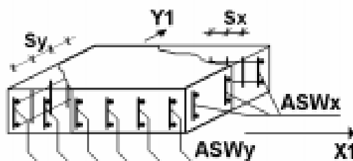
Рисунок 23 – Плита-оболочка
