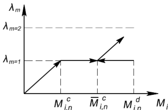
Рисунок 14. Зависимость усилия M_i от параметра внешней нагрузки
