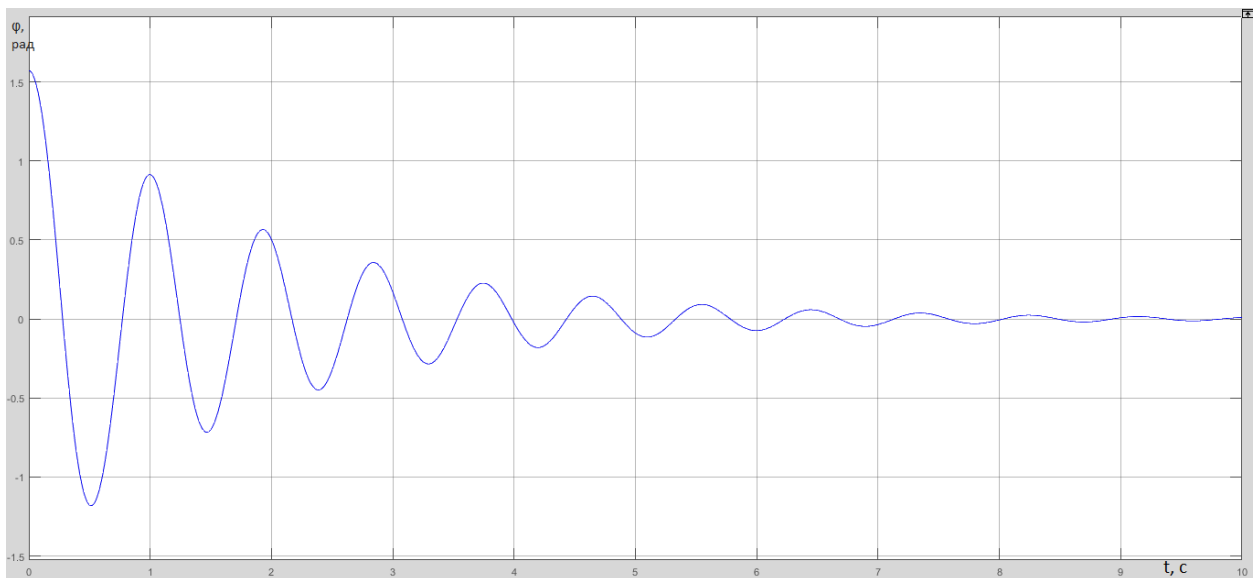
Рис. 13. Результат построения графика изменения угла поворота маятника с помощью блока «Scope»
