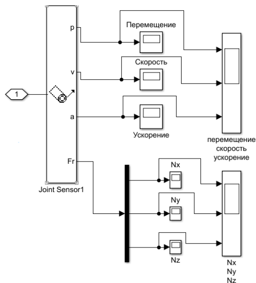
Рис. 4.15 Подсистема «Измерения - ползун»
