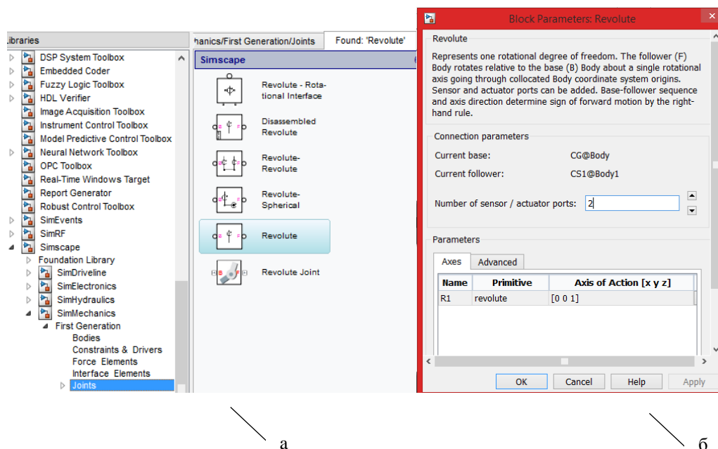
Рис.2.5 Блок Joint Kevolute: а)-расположение в библиотеке, б)-параметры настройки
