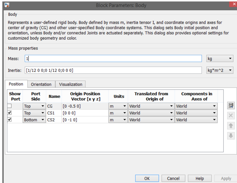
Рис. 1.28 Окно настройки блока «Body»
