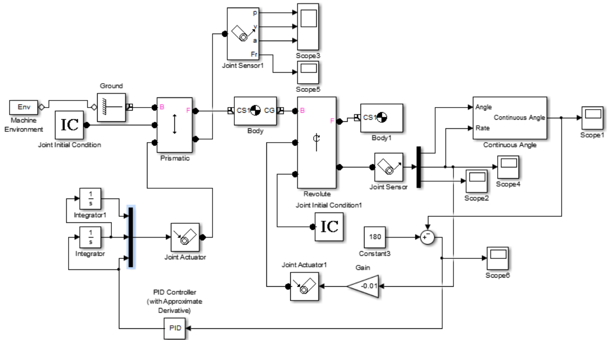
Рис. 2.14 Схема модели ползуна с обращенным маятником
