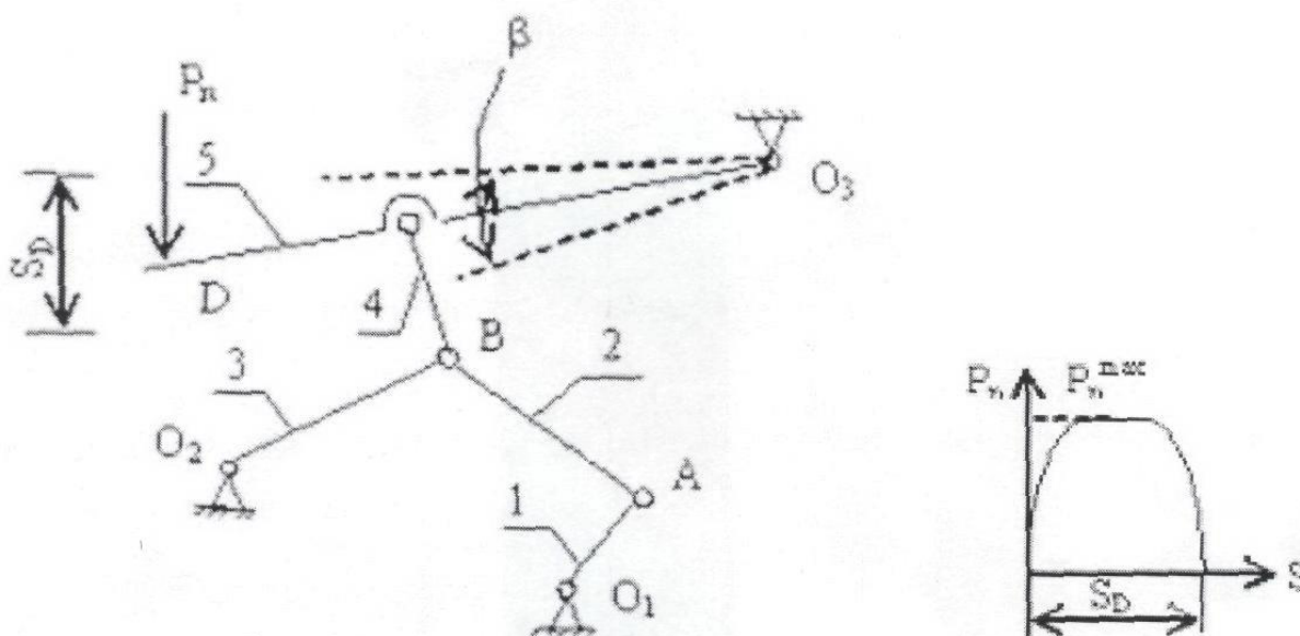
Рис.1. Расчетная схема механизма
