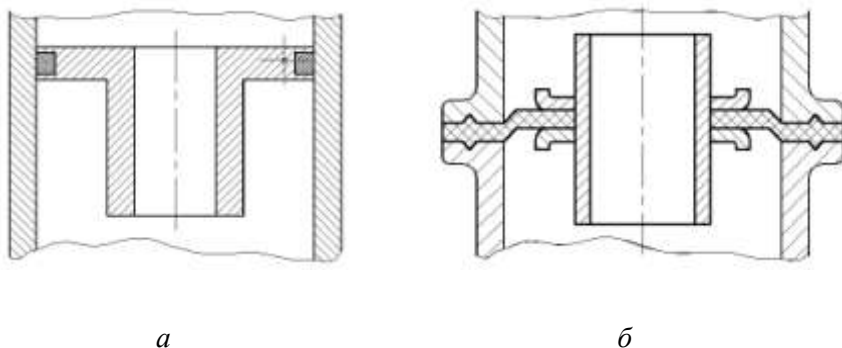
Рисунок 1.8 – Подвижные элементы следящих механизмов: a – поршень; б – мембрана (диафрагма)
