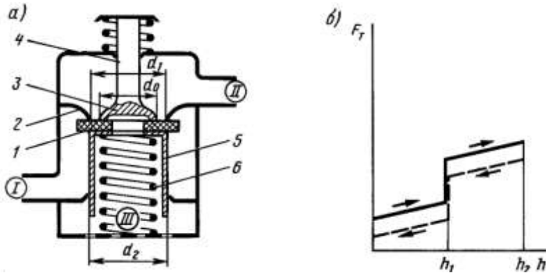
Рисунок 1.3 – Пневмоаппарат с разгруженным клапаном двойного действия: a – расчетная схема; б – статическая характеристика:
