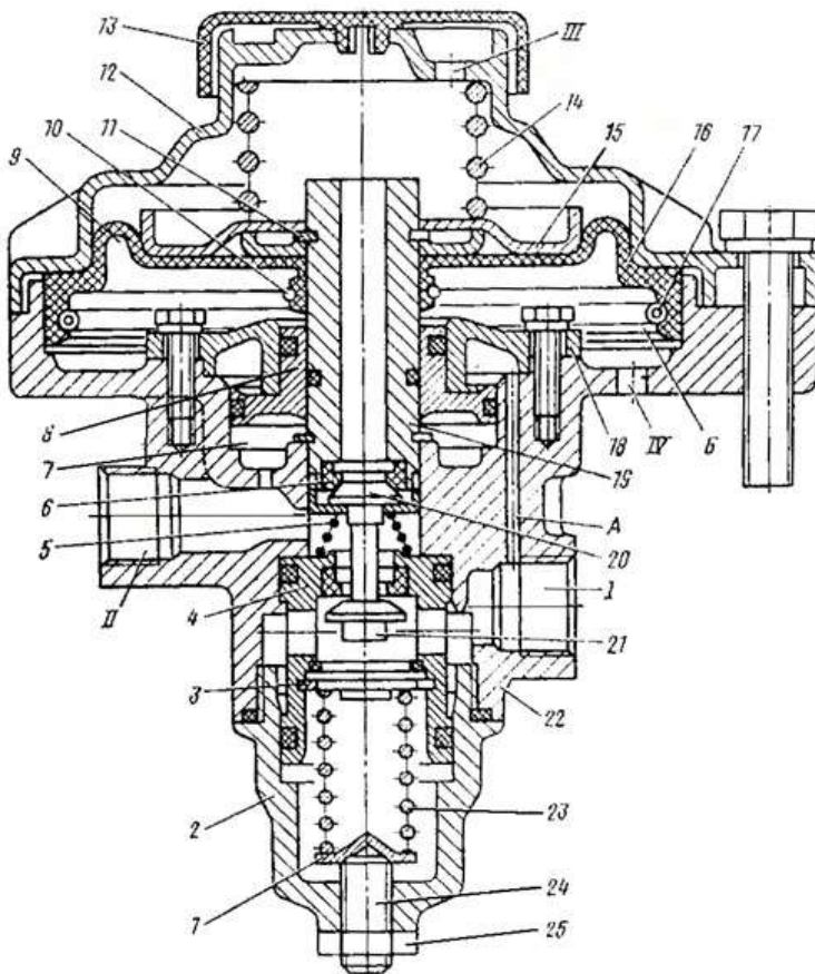
Рисунок 3.5 – Клапан управления тормозами прицепа с однопроводным приводом
