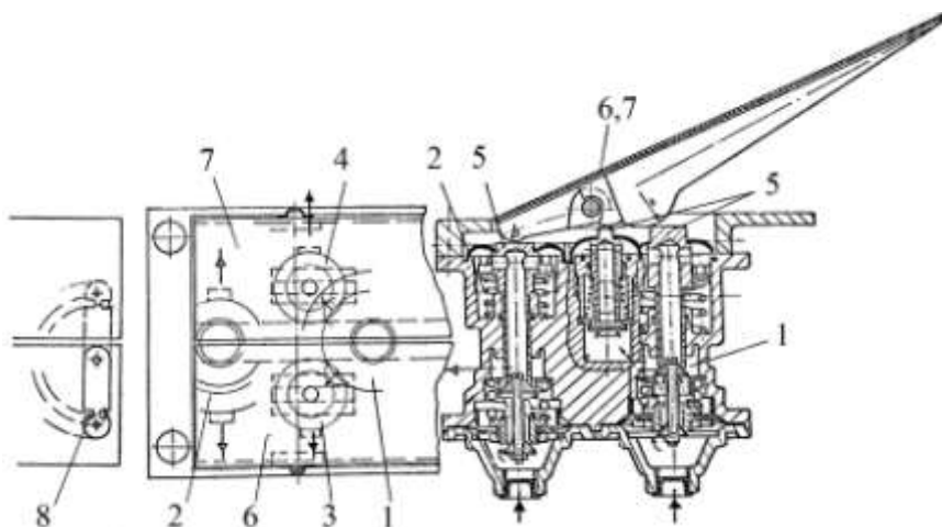
Рисунок 3.13 – Подпедальный комбинированный тормозной кран
