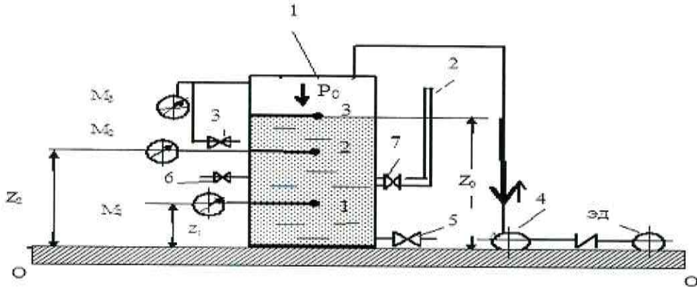
Рис.2 Схема стенда
